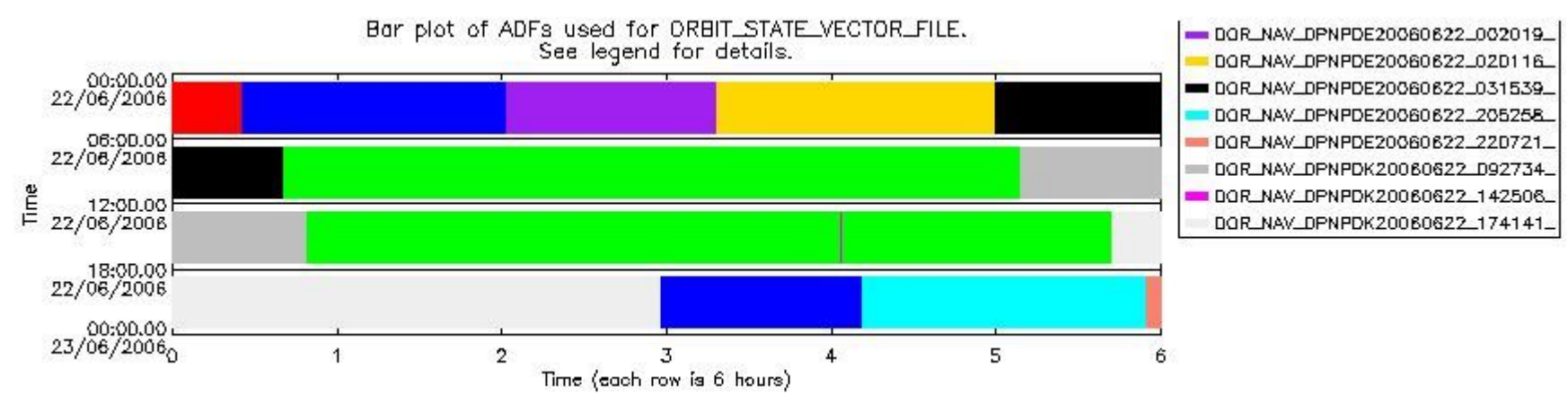
sciamachy_daily_report_level0_PFHS_5_36_N_20060622_6.PNG
