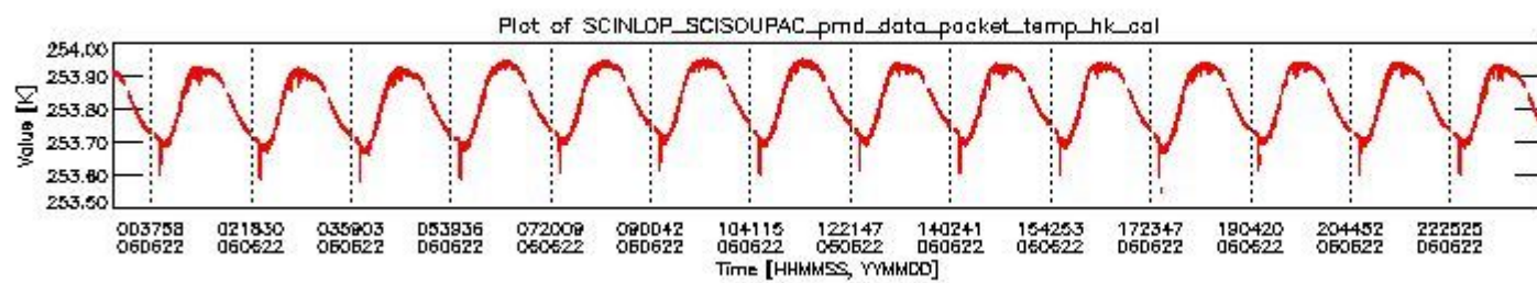
sciamachy_daily_report_level0_PFHS_5_36_N_20060622_3.PNG
