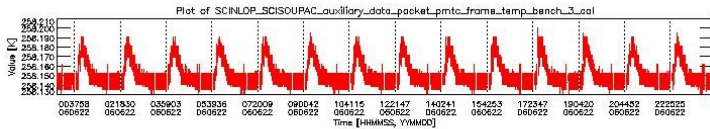
sciamachy_daily_report_level0_PFHS_5_36_N_20060622_2.PNG
