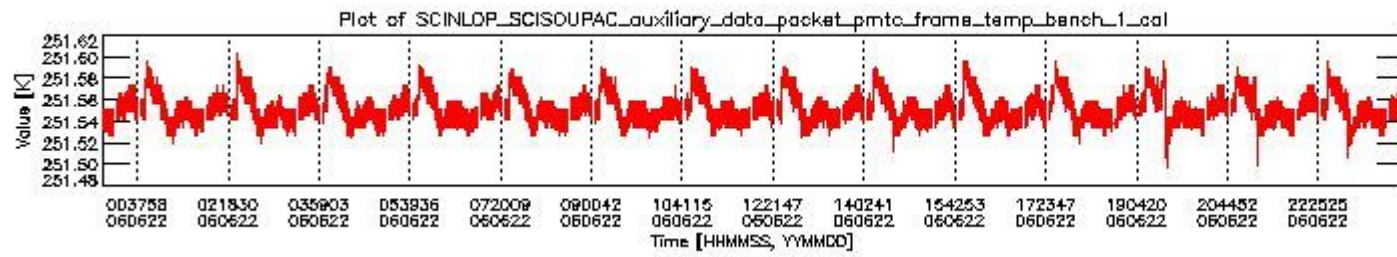
sciamachy_daily_report_level0_PFHS_5_36_N_20060622_0.PNG
