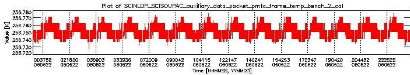
sciamachy_daily_report_level0_PFHS_5_36_N_20060622_1.PNG
