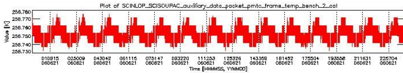
sciamachy_daily_report_level0_PFHS_5_36_N_20060621_1.PNG
