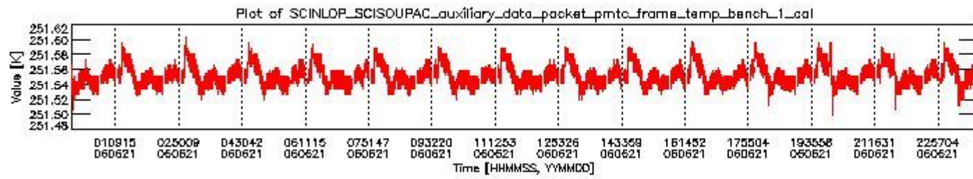
sciamachy_daily_report_level0_PFHS_5_36_N_20060621_0.PNG
