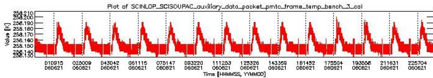
sciamachy_daily_report_level0_PFHS_5_36_N_20060621_2.PNG
