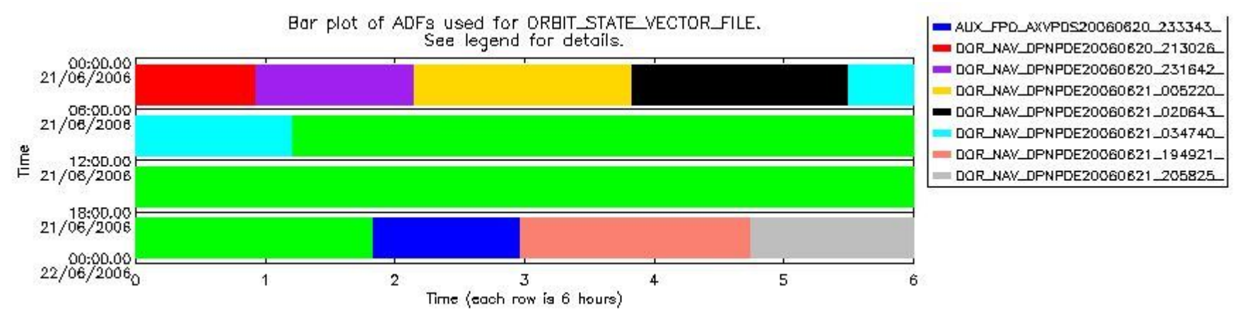
sciamachy_daily_report_level0_PFHS_5_36_N_20060621_6.PNG
