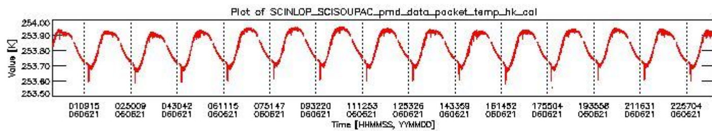
sciamachy_daily_report_level0_PFHS_5_36_N_20060621_3.PNG
