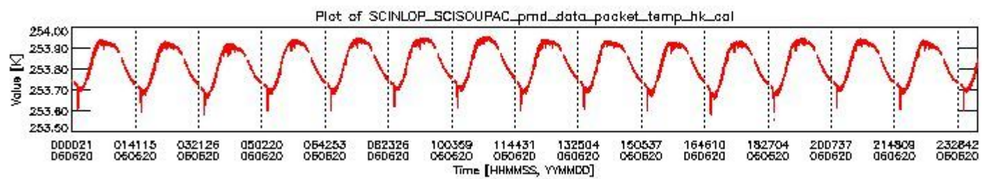
sciamachy_daily_report_level0_PFHS_5_36_N_20060620_3.PNG
