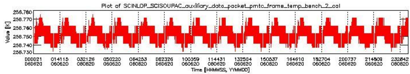
sciamachy_daily_report_level0_PFHS_5_36_N_20060620_1.PNG
