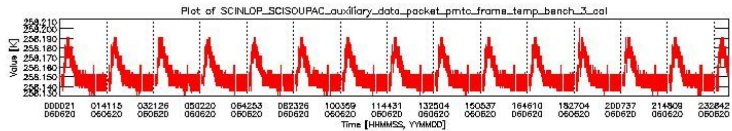
sciamachy_daily_report_level0_PFHS_5_36_N_20060620_2.PNG
