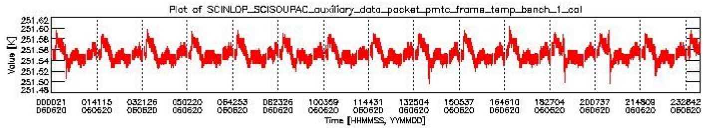
sciamachy_daily_report_level0_PFHS_5_36_N_20060620_0.PNG
