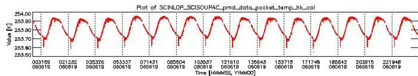
sciamachy_daily_report_level0_PFHS_5_36_N_20060619_3.PNG
