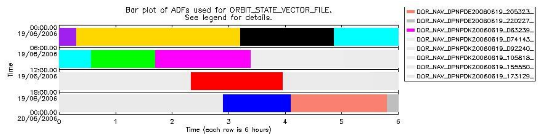
sciamachy_daily_report_level0_PFHS_5_36_N_20060619_6.PNG
