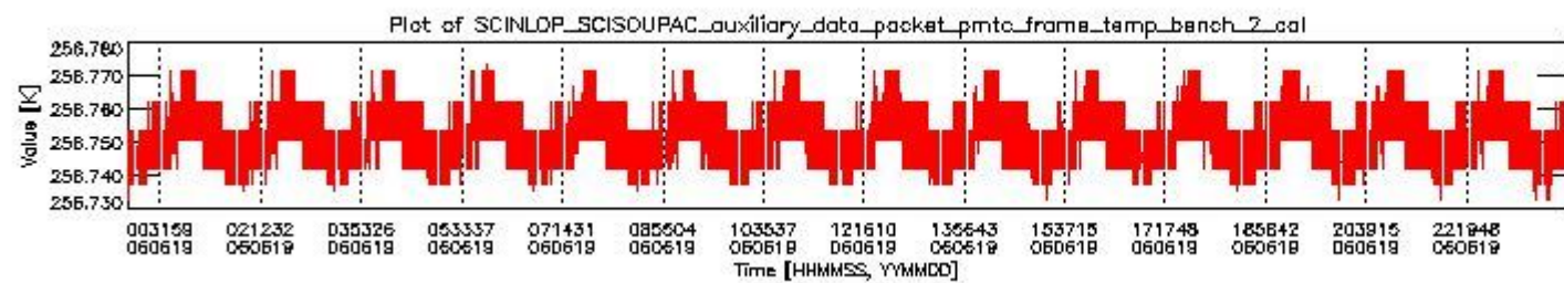
sciamachy_daily_report_level0_PFHS_5_36_N_20060619_1.PNG
