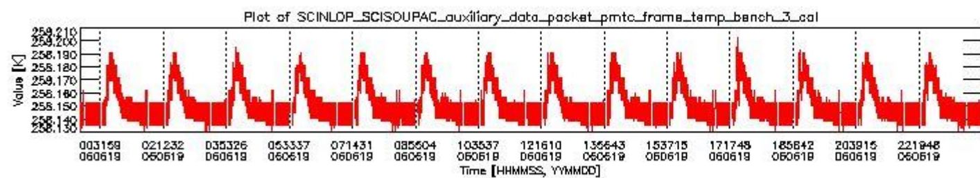
sciamachy_daily_report_level0_PFHS_5_36_N_20060619_2.PNG
