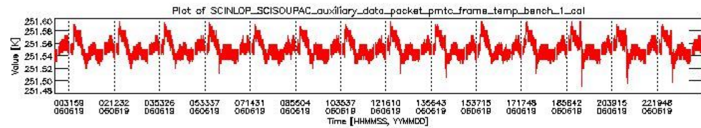
sciamachy_daily_report_level0_PFHS_5_36_N_20060619_0.PNG
