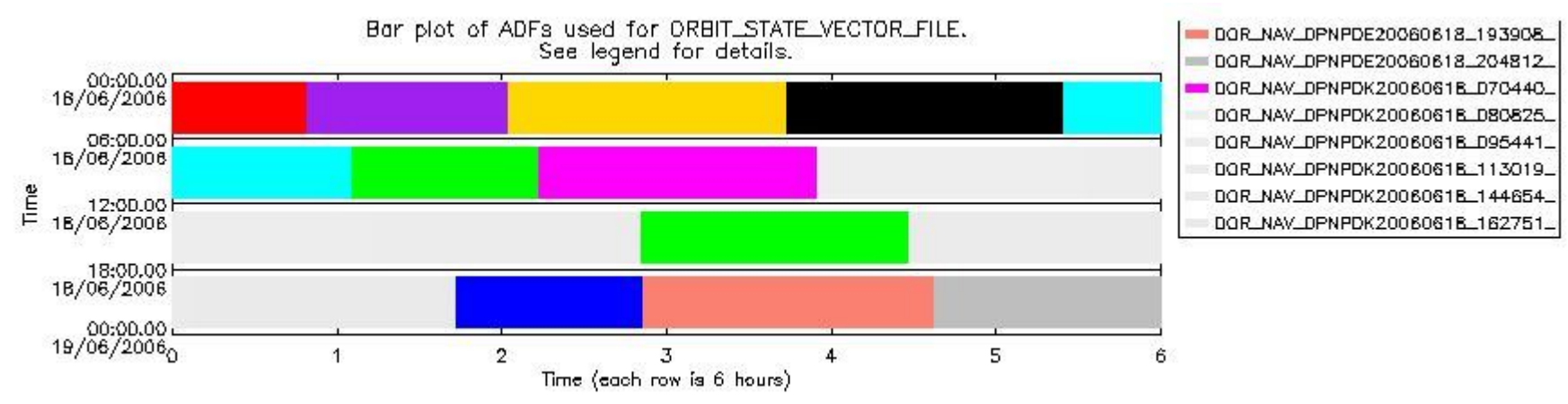
sciamachy_daily_report_level0_PFHS_5_36_N_20060618_6.PNG
