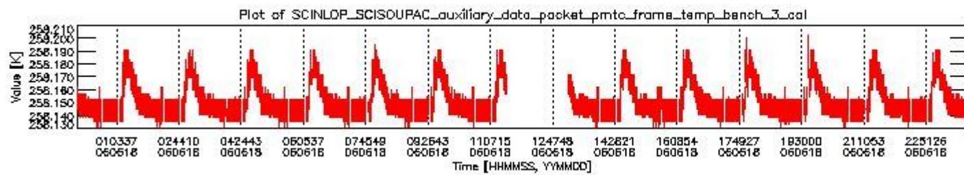
sciamachy_daily_report_level0_PFHS_5_36_N_20060618_2.PNG
