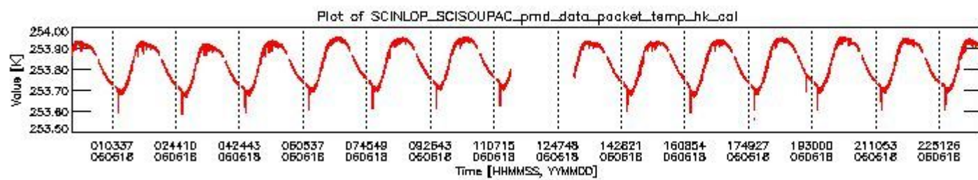
sciamachy_daily_report_level0_PFHS_5_36_N_20060618_3.PNG
