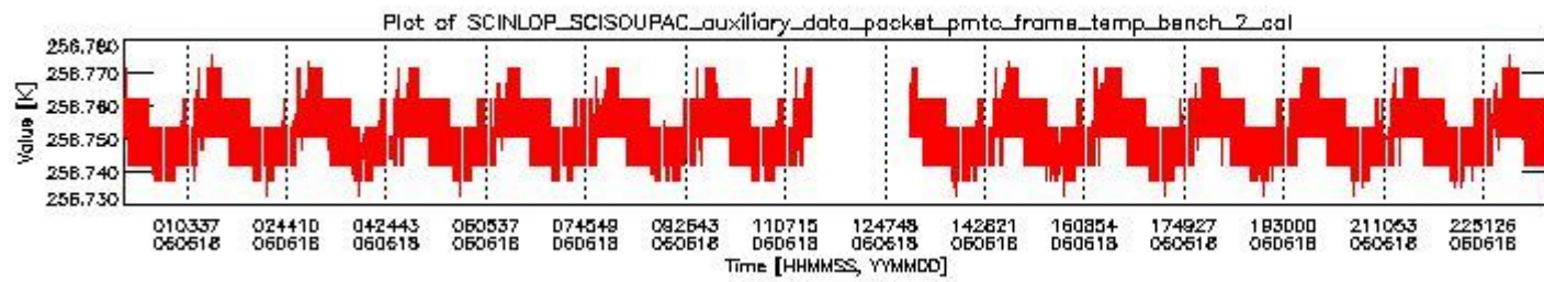
sciamachy_daily_report_level0_PFHS_5_36_N_20060618_1.PNG
