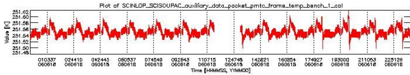
sciamachy_daily_report_level0_PFHS_5_36_N_20060618_0.PNG
