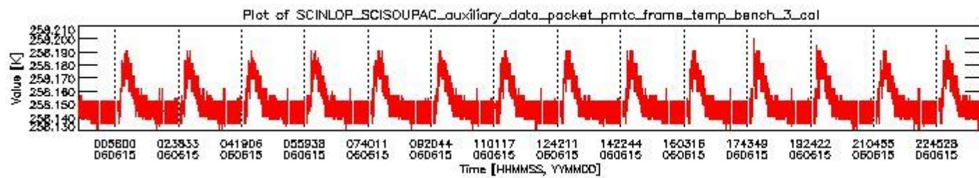
sciamachy_daily_report_level0_PFHS_5_36_N_20060615_2.PNG
