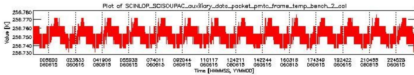
sciamachy_daily_report_level0_PFHS_5_36_N_20060615_1.PNG
