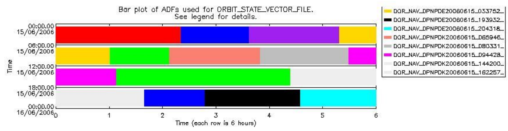
sciamachy_daily_report_level0_PFHS_5_36_N_20060615_6.PNG
