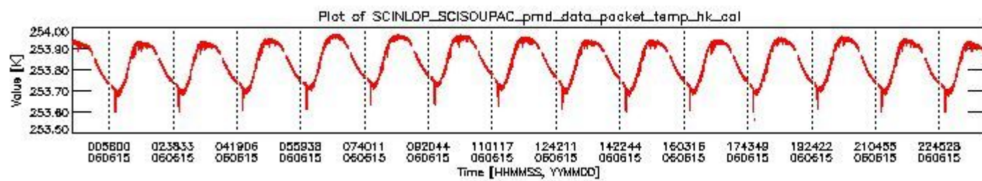
sciamachy_daily_report_level0_PFHS_5_36_N_20060615_3.PNG
