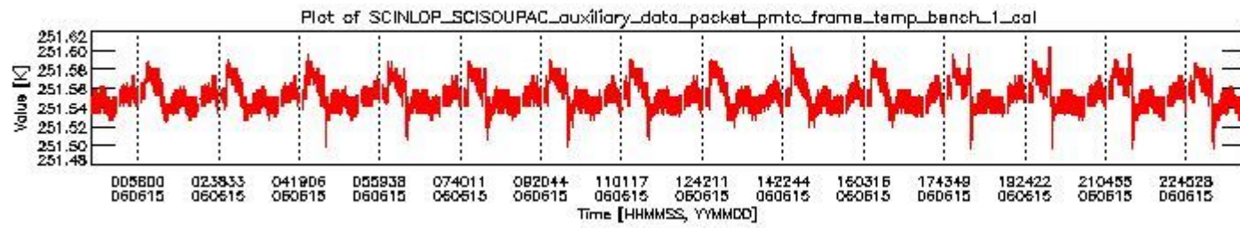
sciamachy_daily_report_level0_PFHS_5_36_N_20060615_0.PNG
