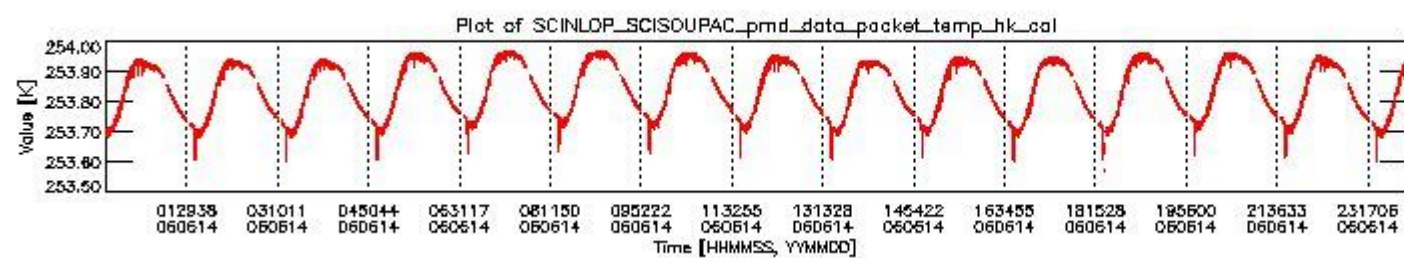
sciamachy_daily_report_level0_PFHS_5_36_N_20060614_3.PNG
