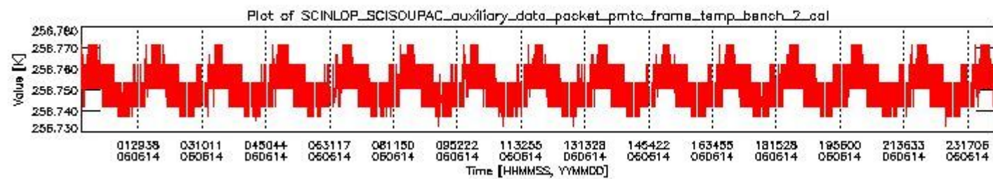
sciamachy_daily_report_level0_PFHS_5_36_N_20060614_1.PNG
