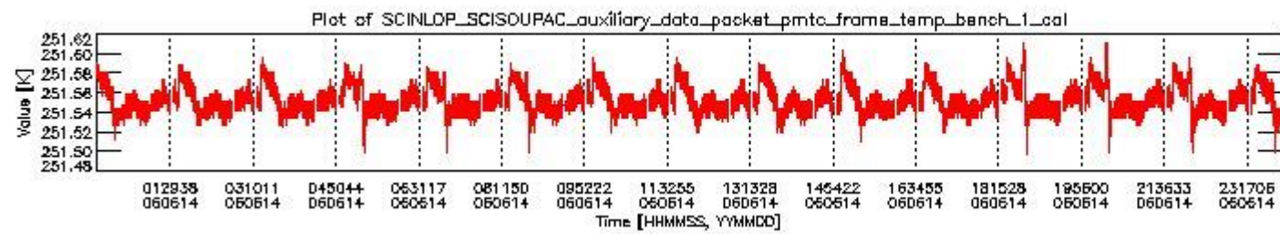
sciamachy_daily_report_level0_PFHS_5_36_N_20060614_0.PNG
