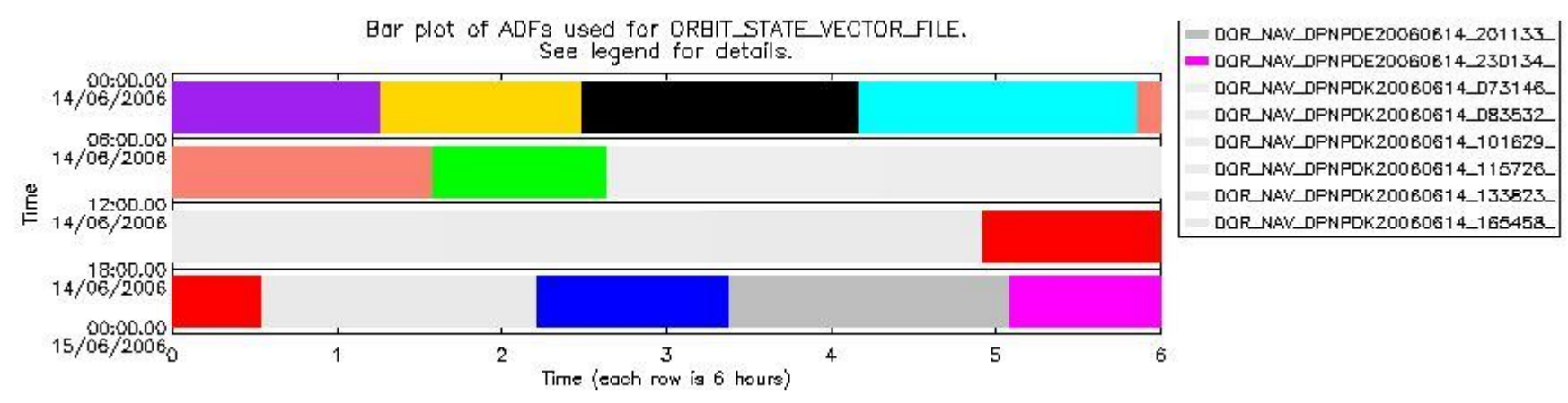
sciamachy_daily_report_level0_PFHS_5_36_N_20060614_6.PNG
