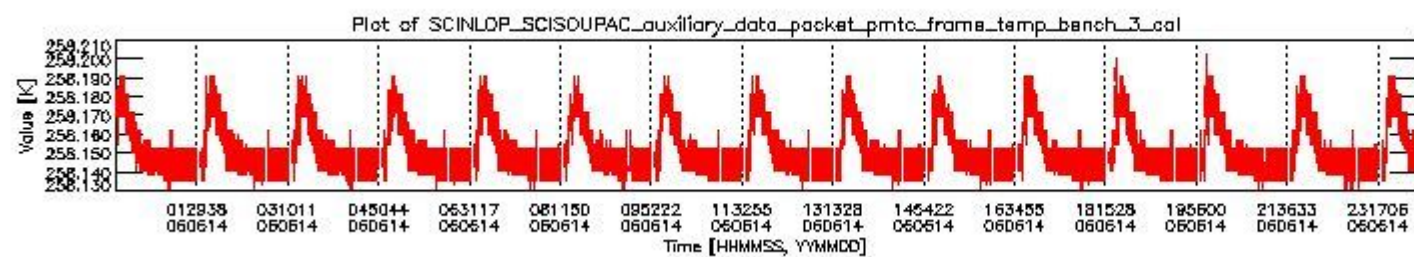
sciamachy_daily_report_level0_PFHS_5_36_N_20060614_2.PNG
