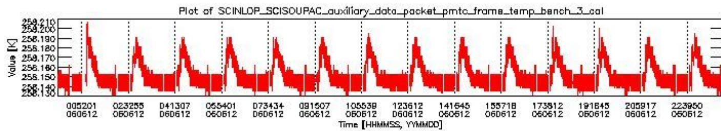
sciamachy_daily_report_level0_PFHS_5_36_N_20060612_2.PNG
