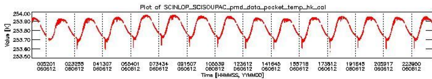
sciamachy_daily_report_level0_PFHS_5_36_N_20060612_3.PNG
