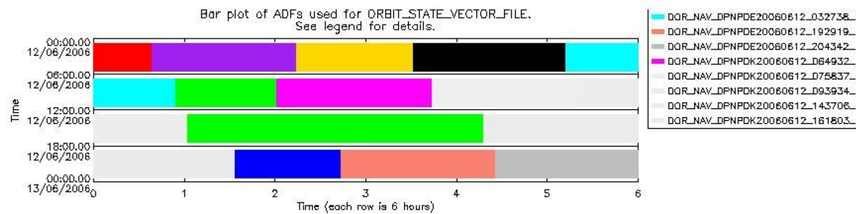
sciamachy_daily_report_level0_PFHS_5_36_N_20060612_6.PNG
