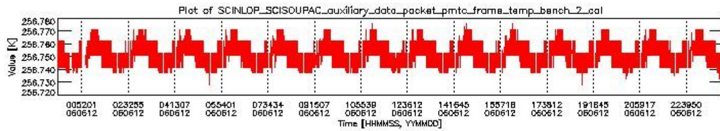
sciamachy_daily_report_level0_PFHS_5_36_N_20060612_1.PNG
