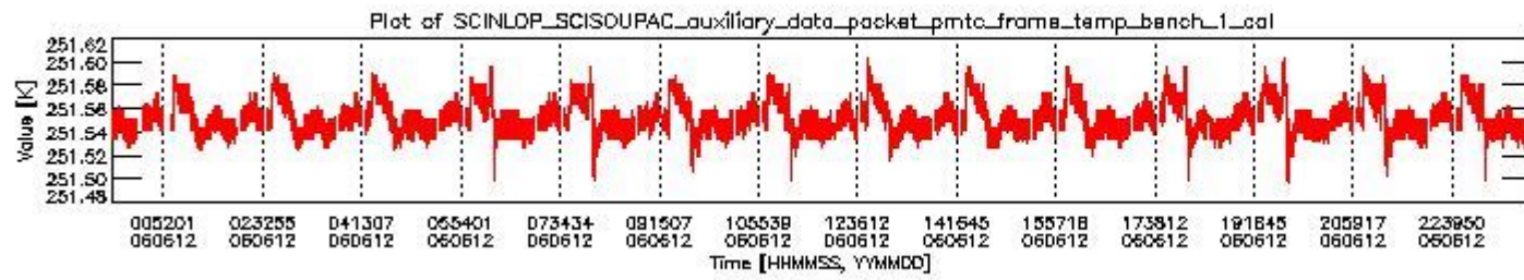
sciamachy_daily_report_level0_PFHS_5_36_N_20060612_0.PNG
