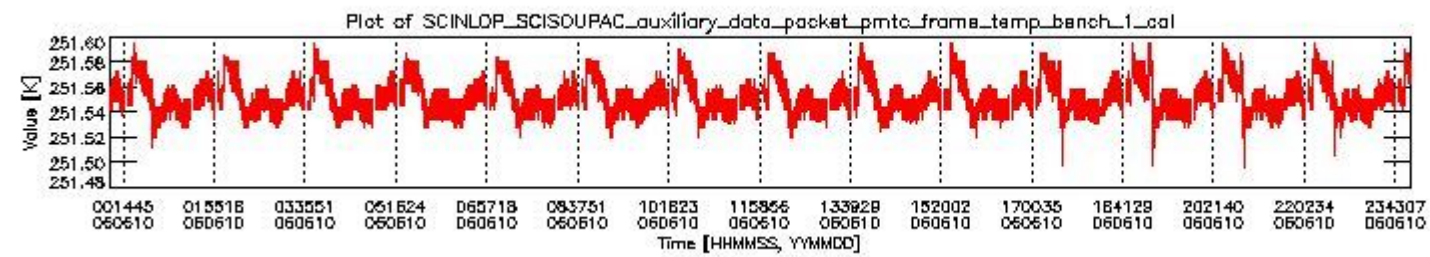
sciamachy_daily_report_level0_PFHS_5_36_N_20060610_0.PNG
