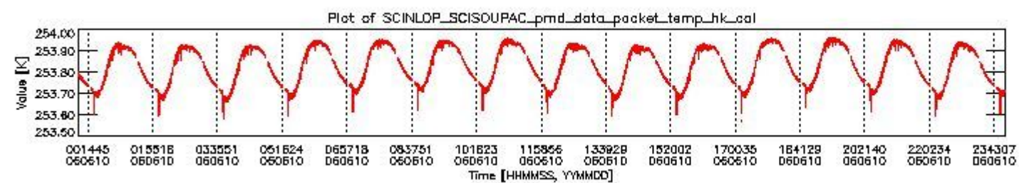
sciamachy_daily_report_level0_PFHS_5_36_N_20060610_3.PNG
