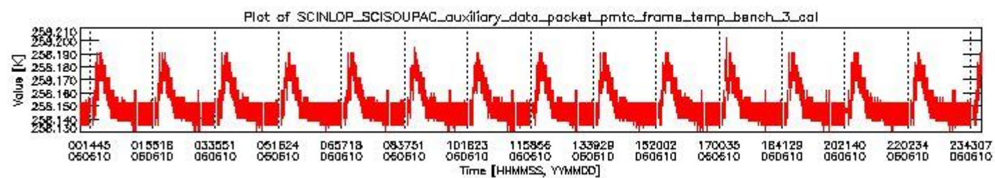
sciamachy_daily_report_level0_PFHS_5_36_N_20060610_2.PNG
