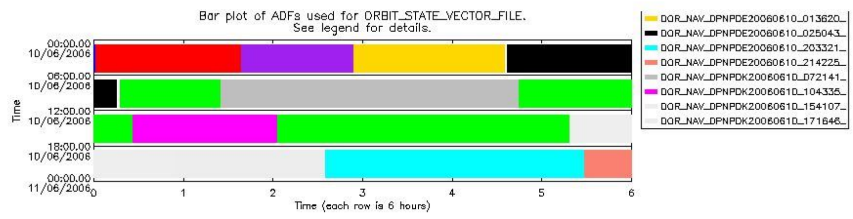
sciamachy_daily_report_level0_PFHS_5_36_N_20060610_6.PNG
