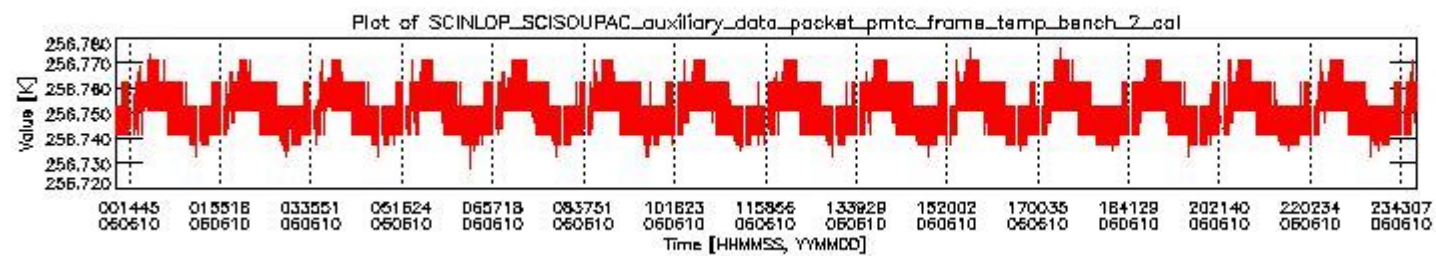
sciamachy_daily_report_level0_PFHS_5_36_N_20060610_1.PNG
