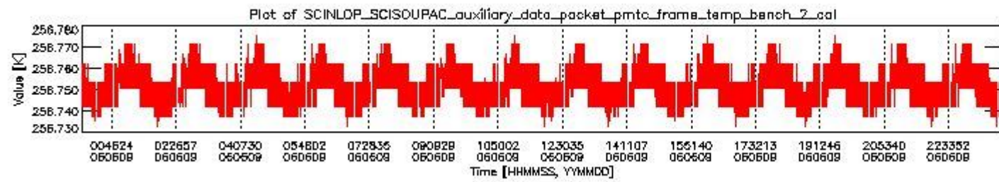
sciamachy_daily_report_level0_PFHS_5_36_N_20060609_1.PNG
