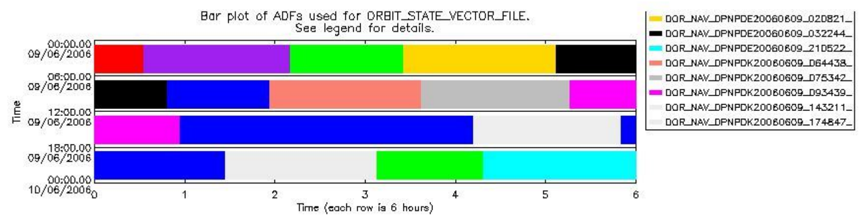
sciamachy_daily_report_level0_PFHS_5_36_N_20060609_6.PNG
