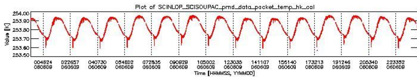
sciamachy_daily_report_level0_PFHS_5_36_N_20060609_3.PNG
