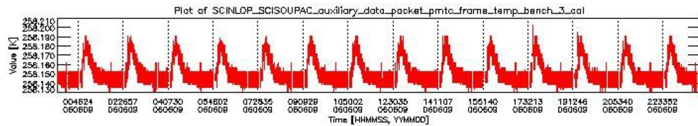
sciamachy_daily_report_level0_PFHS_5_36_N_20060609_2.PNG
