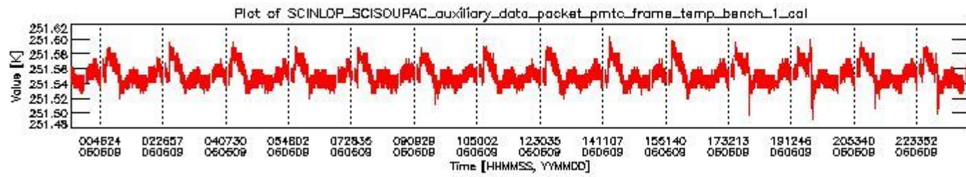
sciamachy_daily_report_level0_PFHS_5_36_N_20060609_0.PNG
