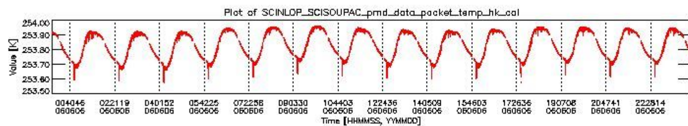
sciamachy_daily_report_level0_PFHS_5_36_N_20060606_3.PNG
