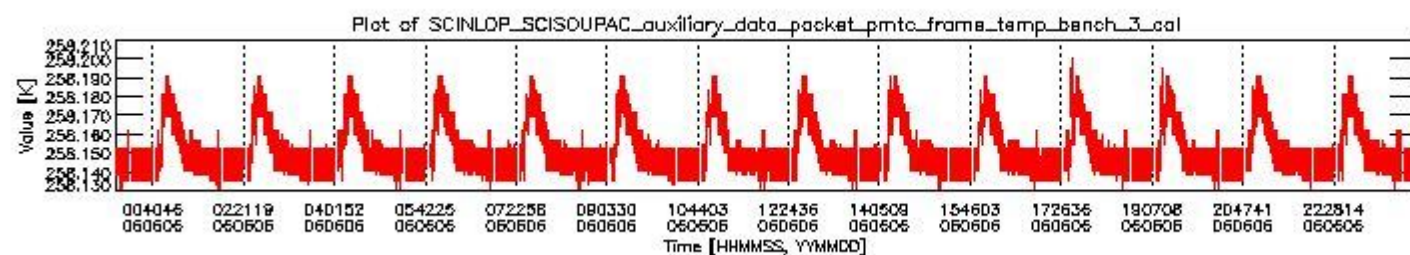
sciamachy_daily_report_level0_PFHS_5_36_N_20060606_2.PNG
