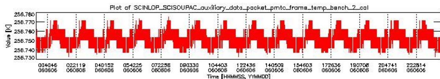
sciamachy_daily_report_level0_PFHS_5_36_N_20060606_1.PNG
