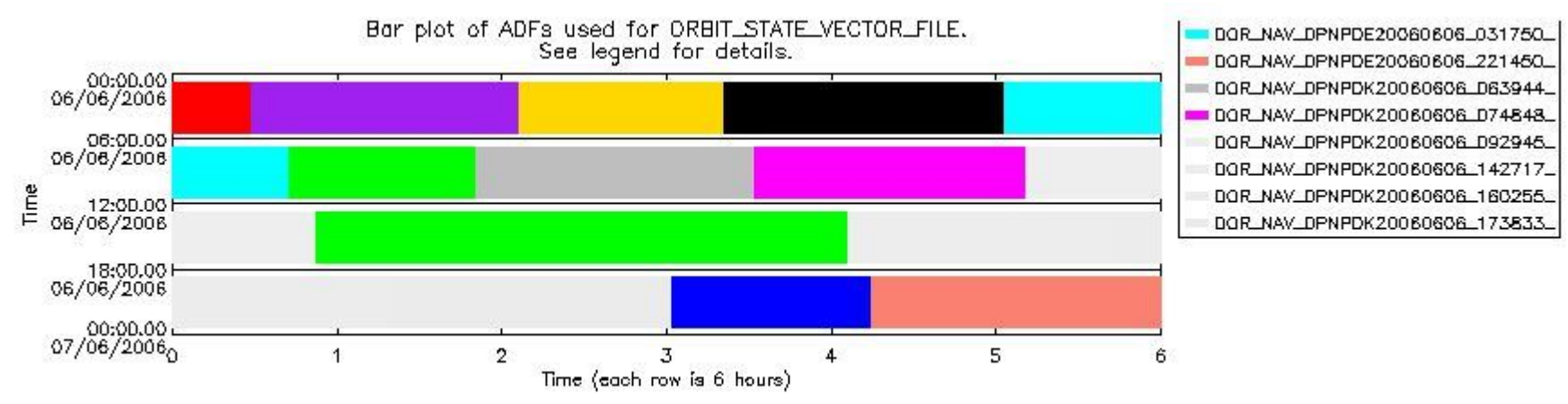
sciamachy_daily_report_level0_PFHS_5_36_N_20060606_6.PNG
