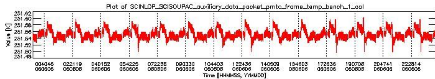
sciamachy_daily_report_level0_PFHS_5_36_N_20060606_0.PNG
