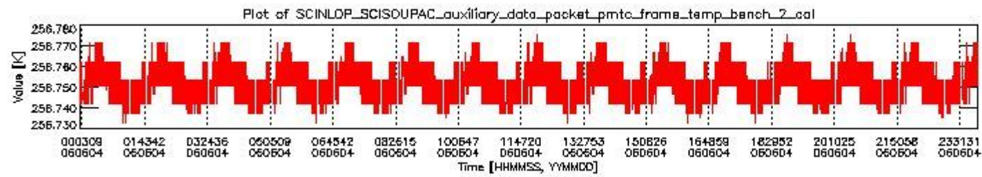
sciamachy_daily_report_level0_PFHS_5_36_N_20060604_1.PNG
