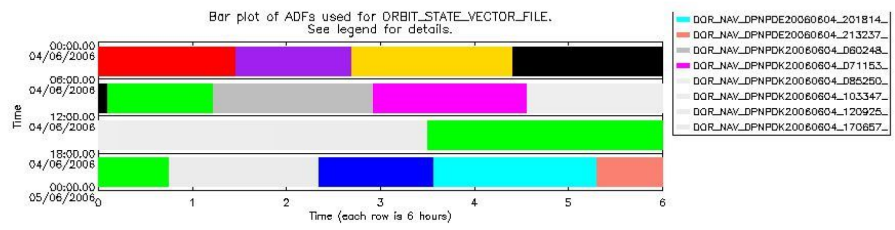
sciamachy_daily_report_level0_PFHS_5_36_N_20060604_6.PNG
