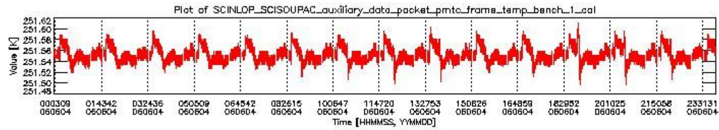
sciamachy_daily_report_level0_PFHS_5_36_N_20060604_0.PNG
