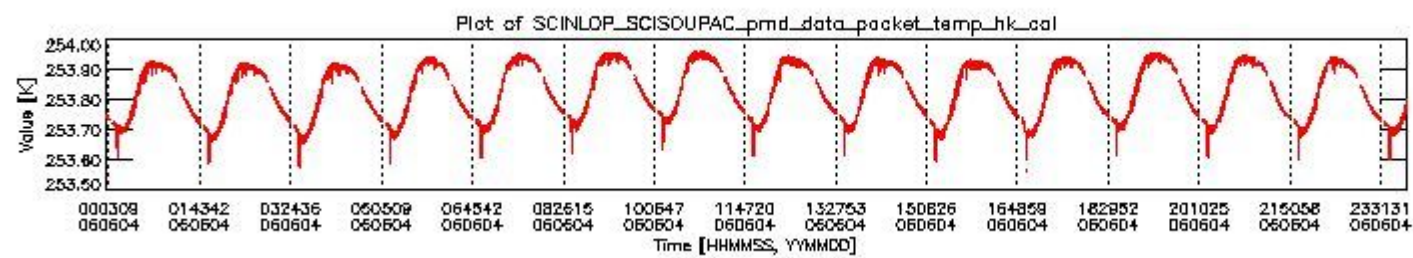
sciamachy_daily_report_level0_PFHS_5_36_N_20060604_3.PNG
