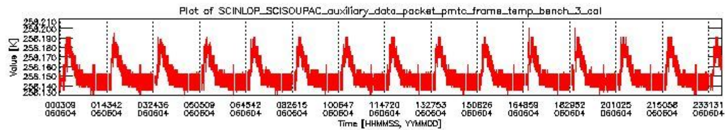
sciamachy_daily_report_level0_PFHS_5_36_N_20060604_2.PNG
