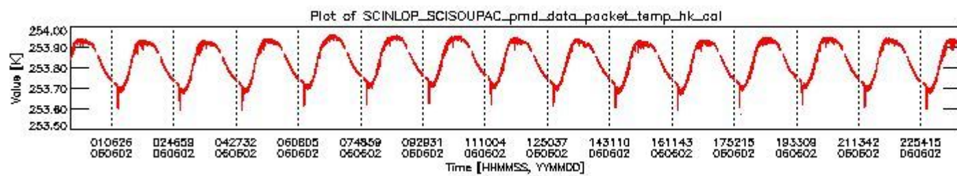
sciamachy_daily_report_level0_PFHS_5_36_N_20060602_3.PNG
