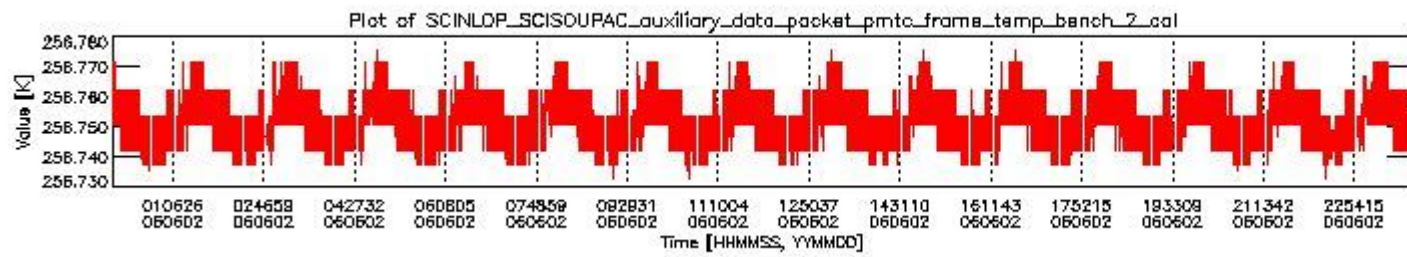
sciamachy_daily_report_level0_PFHS_5_36_N_20060602_1.PNG
