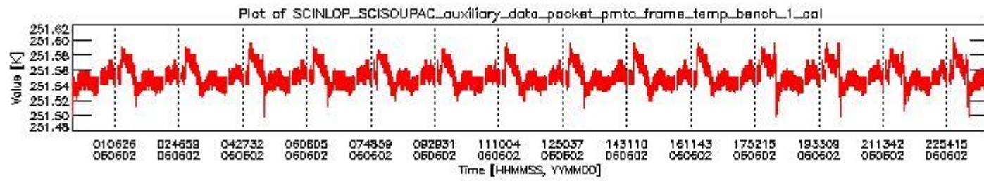
sciamachy_daily_report_level0_PFHS_5_36_N_20060602_0.PNG
