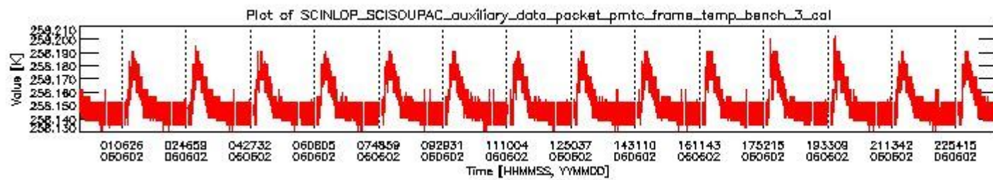
sciamachy_daily_report_level0_PFHS_5_36_N_20060602_2.PNG
