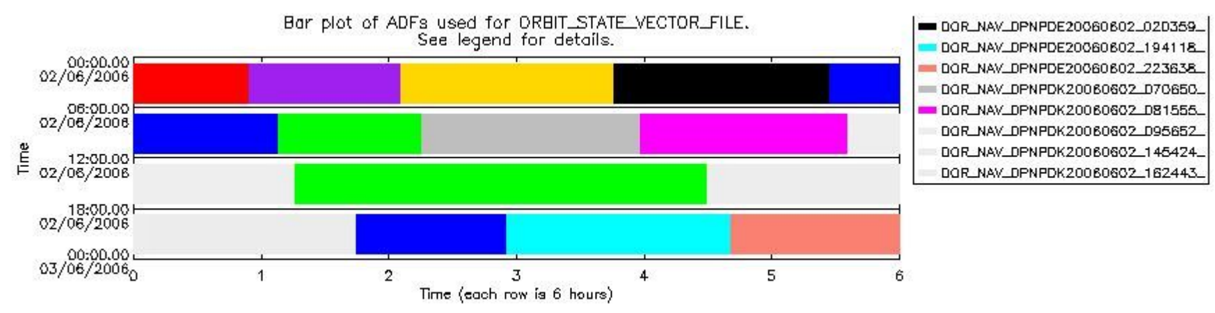
sciamachy_daily_report_level0_PFHS_5_36_N_20060602_6.PNG
