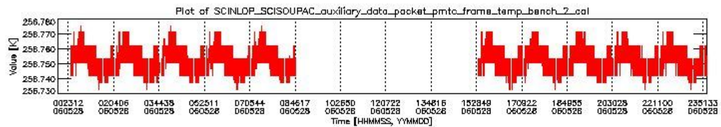
sciamachy_daily_report_level0_PFHS_5_36_N_20060528_1.PNG
