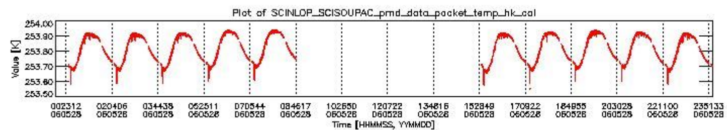
sciamachy_daily_report_level0_PFHS_5_36_N_20060528_3.PNG
