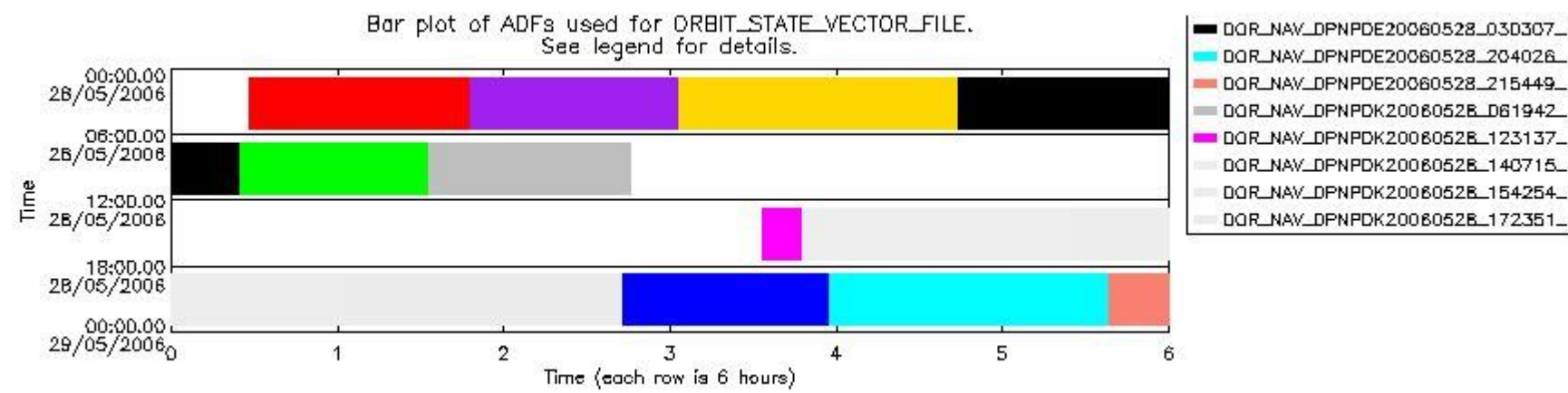
sciamachy_daily_report_level0_PFHS_5_36_N_20060528_6.PNG
