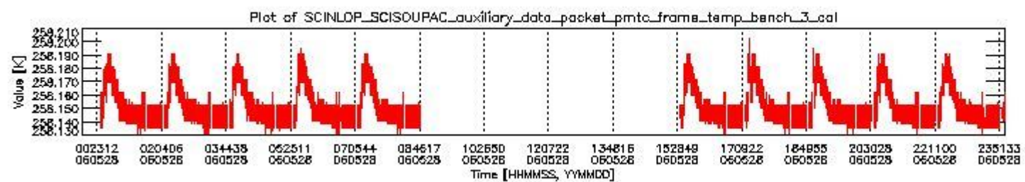
sciamachy_daily_report_level0_PFHS_5_36_N_20060528_2.PNG
