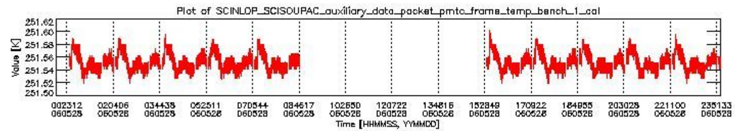
sciamachy_daily_report_level0_PFHS_5_36_N_20060528_0.PNG
