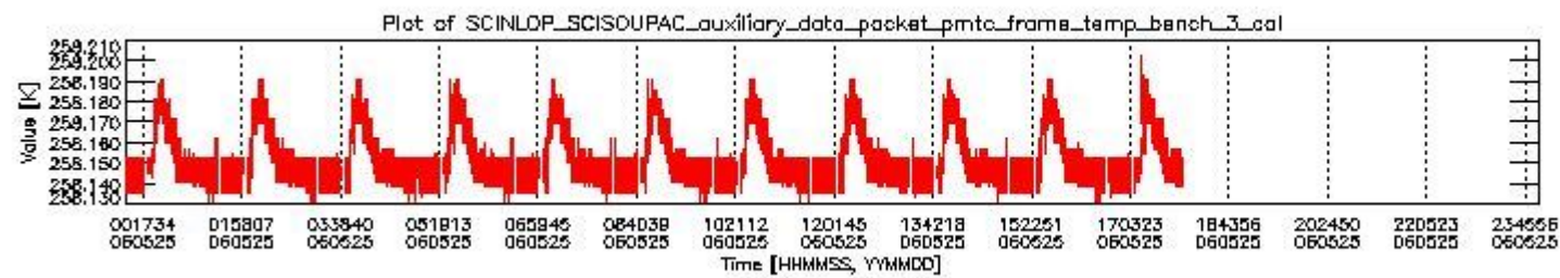
sciamachy_daily_report_level0_PFHS_5_36_N_20060525_2.PNG
