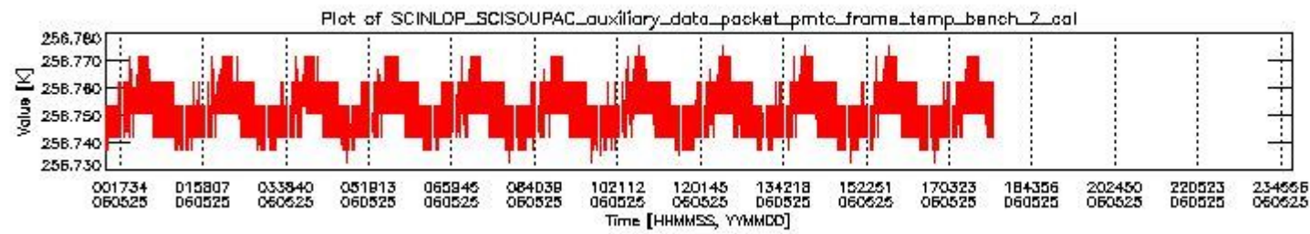
sciamachy_daily_report_level0_PFHS_5_36_N_20060525_1.PNG
