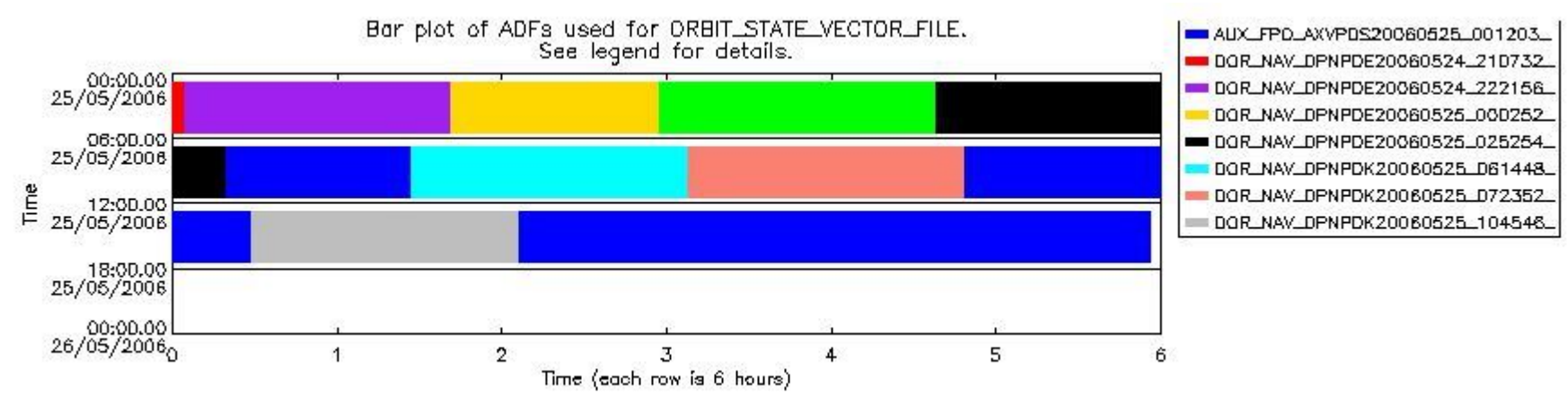
sciamachy_daily_report_level0_PFHS_5_36_N_20060525_6.PNG
