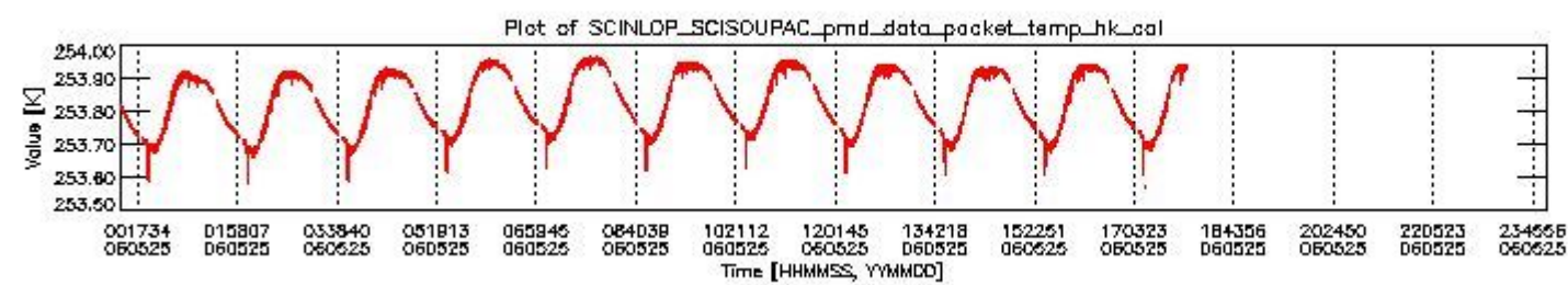
sciamachy_daily_report_level0_PFHS_5_36_N_20060525_3.PNG
