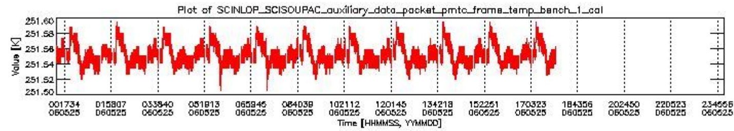
sciamachy_daily_report_level0_PFHS_5_36_N_20060525_0.PNG
