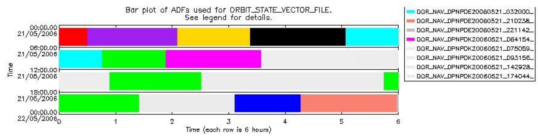
sciamachy_daily_report_level0_PFHS_5_36_N_20060521_6.PNG
