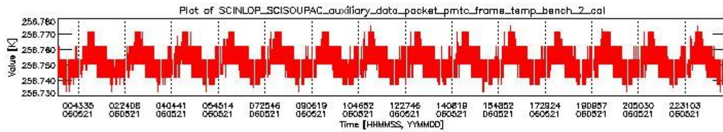
sciamachy_daily_report_level0_PFHS_5_36_N_20060521_1.PNG
