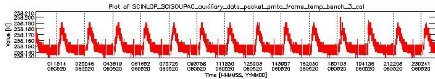
sciamachy_daily_report_level0_PFHS_5_36_N_20060520_2.PNG
