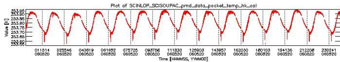
sciamachy_daily_report_level0_PFHS_5_36_N_20060520_3.PNG
