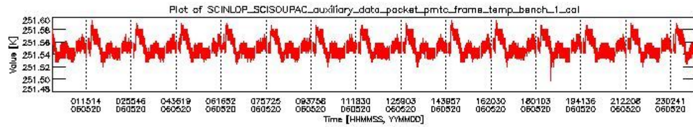
sciamachy_daily_report_level0_PFHS_5_36_N_20060520_0.PNG
