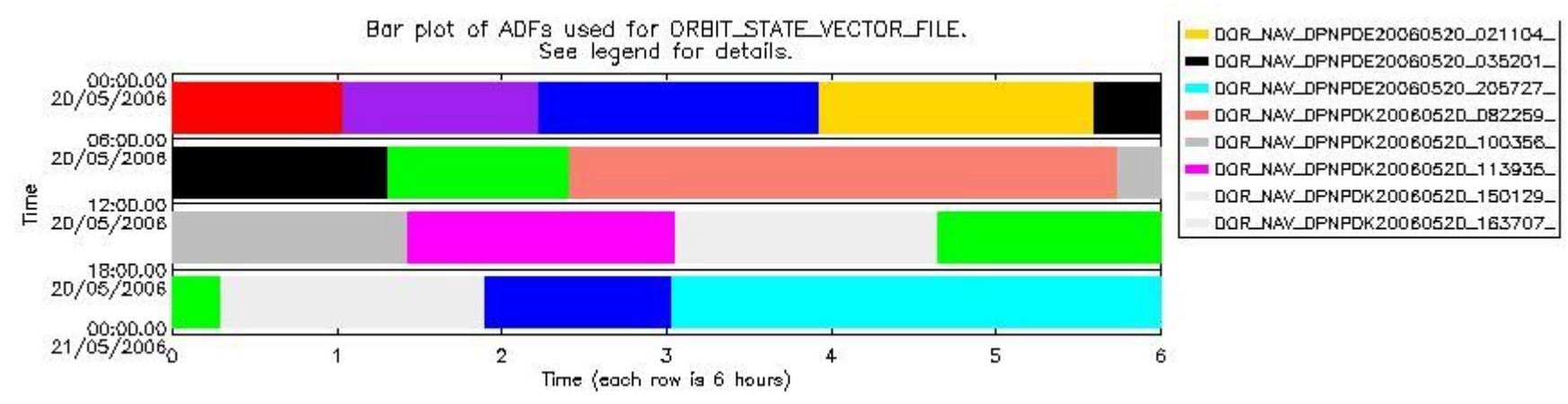
sciamachy_daily_report_level0_PFHS_5_36_N_20060520_6.PNG
