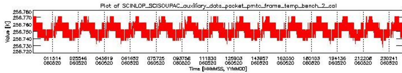
sciamachy_daily_report_level0_PFHS_5_36_N_20060520_1.PNG
