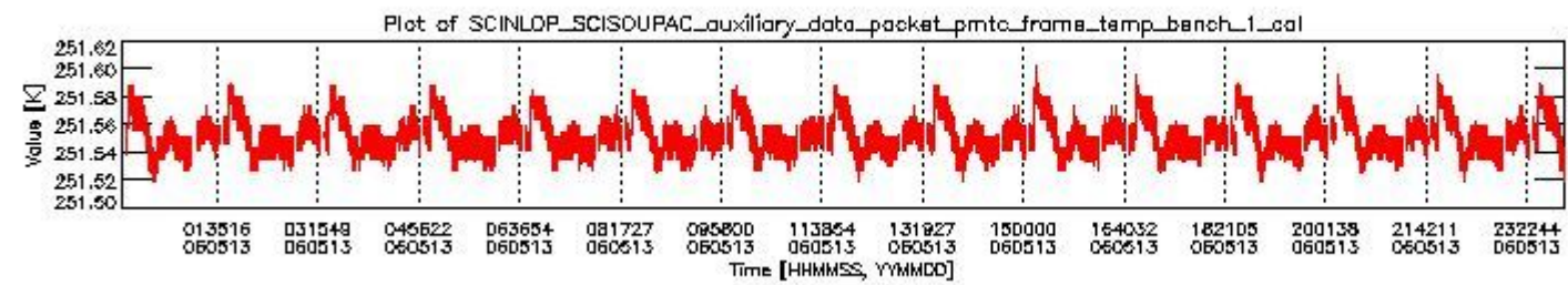
sciamachy_daily_report_level0_PFH5_5_36_N_20060513_0.PNG
