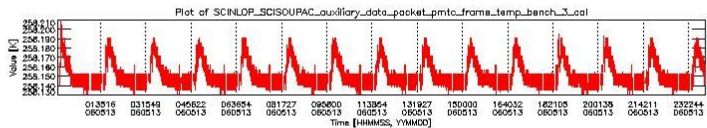
sciamachy_daily_report_level0_PFH5_5_36_N_20060513_2.PNG
