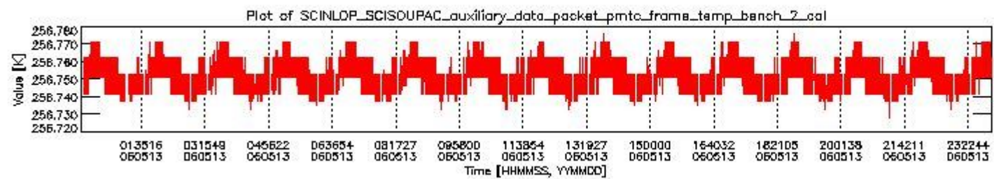
sciamachy_daily_report_level0_PFH5_5_36_N_20060513_1.PNG
