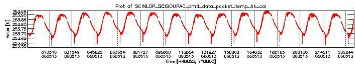
sciamachy_daily_report_level0_PFH5_5_36_N_20060513_3.PNG
