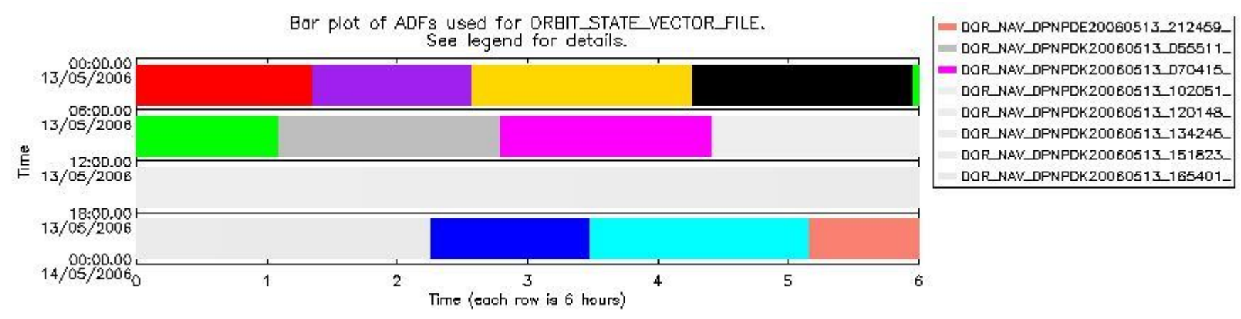
sciamachy_daily_report_level0_PFHS_5_36_N_20060513_6.PNG
