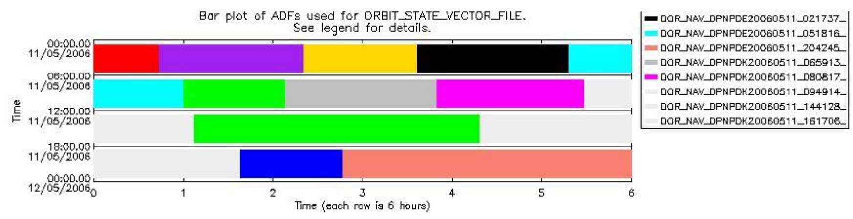
sciamachy_daily_report_level0_PFHS_5_36_N_20060511_6.PNG
