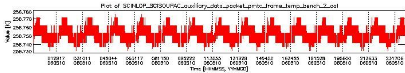
sciamachy_daily_report_level0_PFHS_5_36_N_20060510_1.PNG
