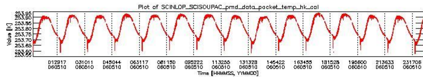
sciamachy_daily_report_level0_PFHS_5_36_N_20060510_3.PNG
