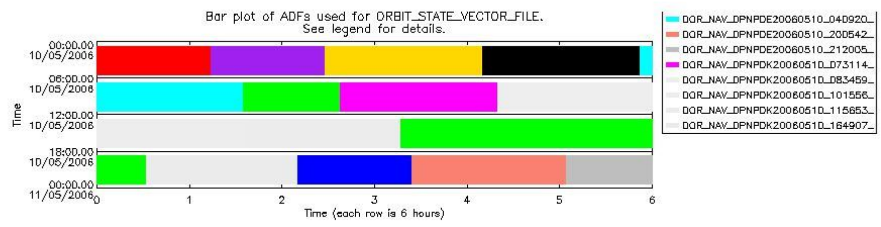
sciamachy_daily_report_level0_PFHS_5_36_N_20060510_6.PNG
