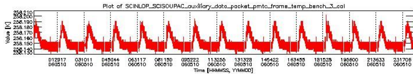
sciamachy_daily_report_level0_PFHS_5_36_N_20060510_2.PNG
