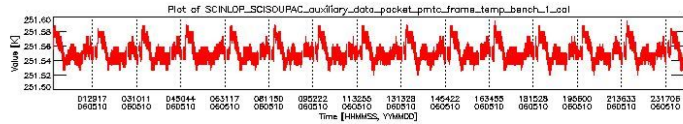
sciamachy_daily_report_level0_PFHS_5_36_N_20060510_0.PNG
