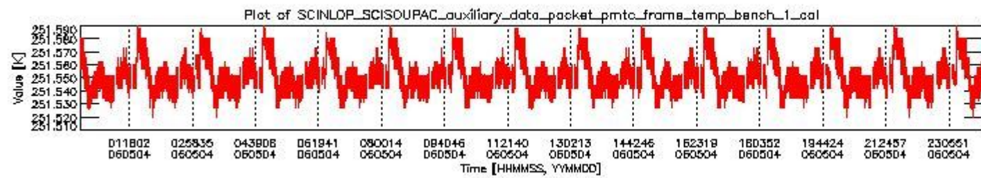
sciamachy_daily_report_level0_PFHS_5_36_N_20060504_0.PNG
