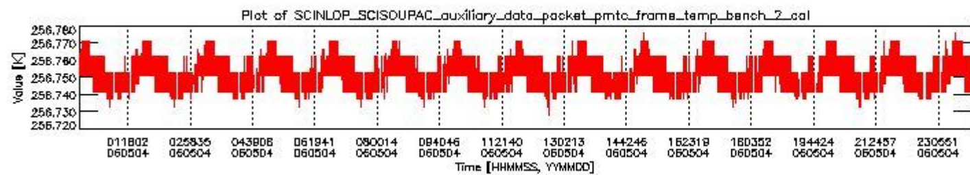
sciamachy_daily_report_level0_PFHS_5_36_N_20060504_1.PNG
