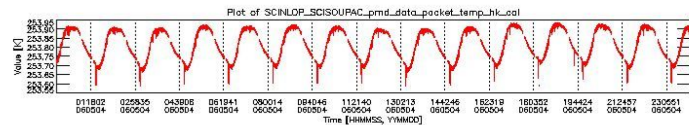
sciamachy_daily_report_level0_PFHS_5_36_N_20060504_3.PNG
