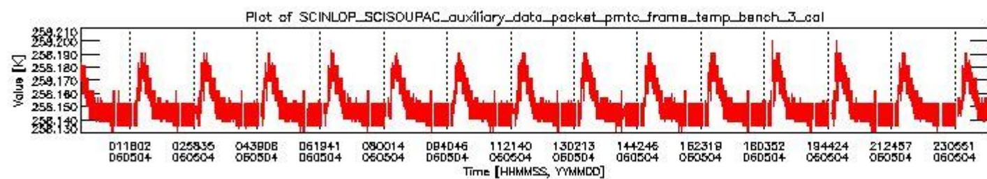
sciamachy_daily_report_level0_PFHS_5_36_N_20060504_2.PNG
