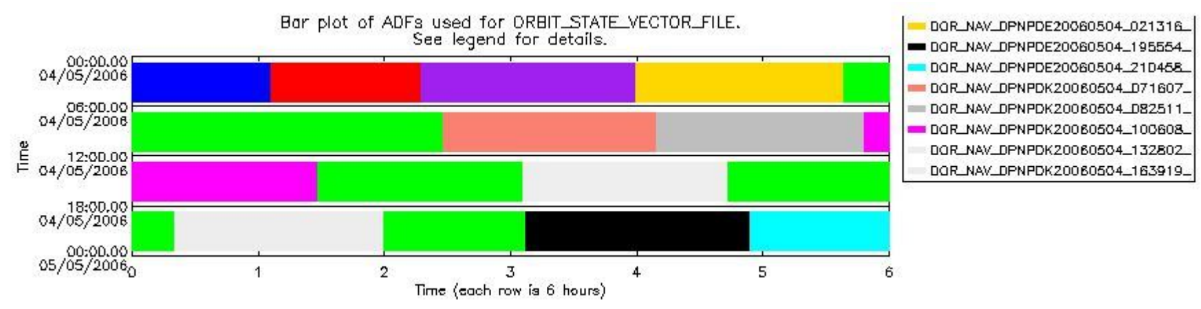
sciamachy_daily_report_level0_PFHS_5_36_N_20060504_6.PNG
