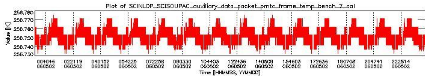
sciamachy_daily_report_level0_PFHS_5_36_N_20060502_1.PNG
