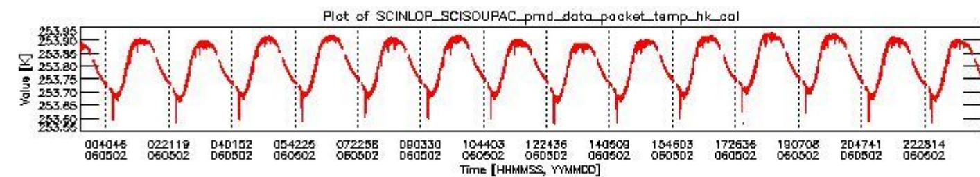
sciamachy_daily_report_level0_PFHS_5_36_N_20060502_3.PNG
