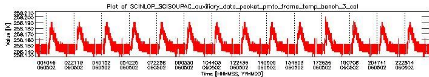
sciamachy_daily_report_level0_PFHS_5_36_N_20060502_2.PNG
