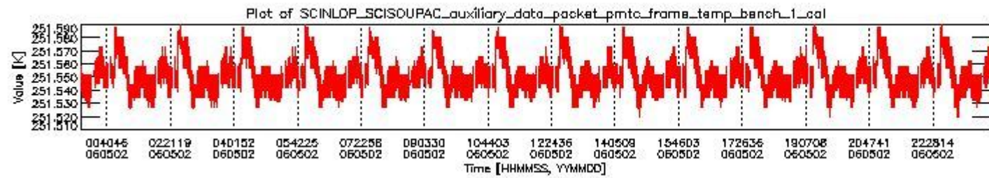
sciamachy_daily_report_level0_PFHS_5_36_N_20060502_0.PNG
