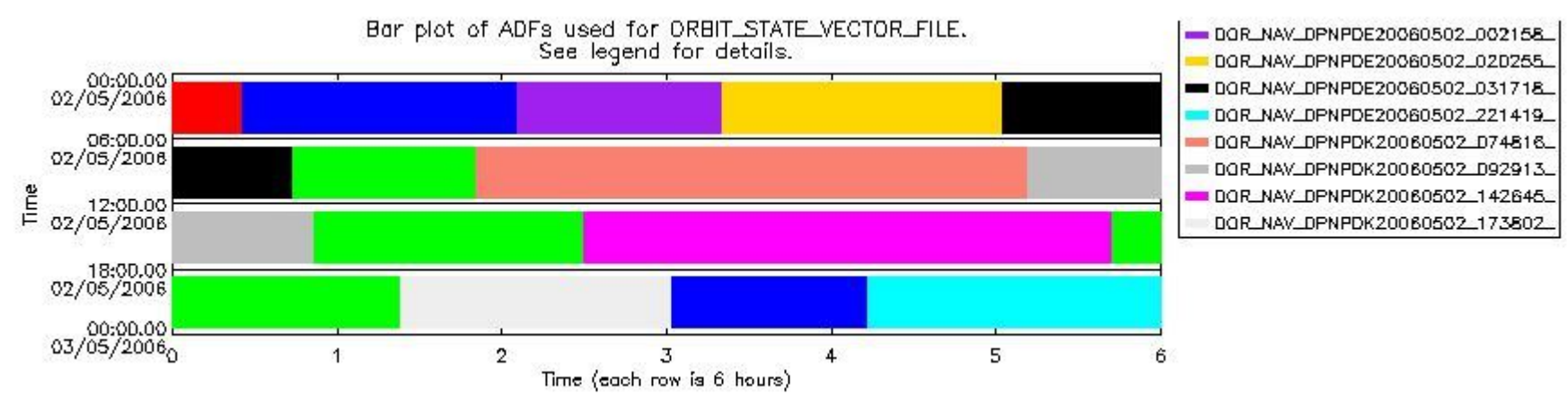
sciamachy_daily_report_level0_PFHS_5_36_N_20060502_6.PNG
