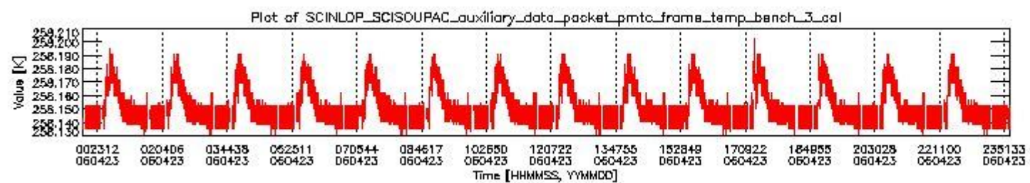
sciamachy_daily_report_level0_PFHS_5_36_N_20060423_2.PNG
