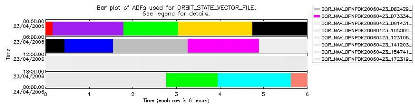
sciamachy_daily_report_level0_PFHS_5_36_N_20060423_6.PNG
