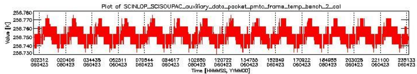
sciamachy_daily_report_level0_PFHS_5_36_N_20060423_1.PNG
