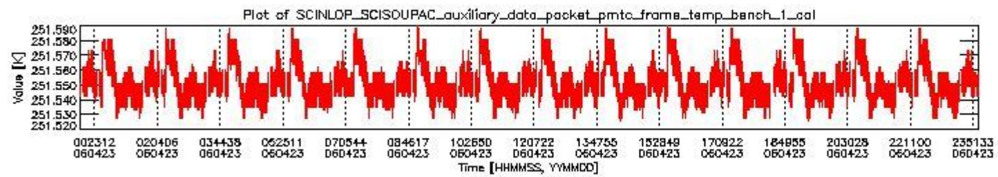
sciamachy_daily_report_level0_PFHS_5_36_N_20060423_0.PNG
