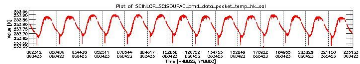
sciamachy_daily_report_level0_PFHS_5_36_N_20060423_3.PNG
