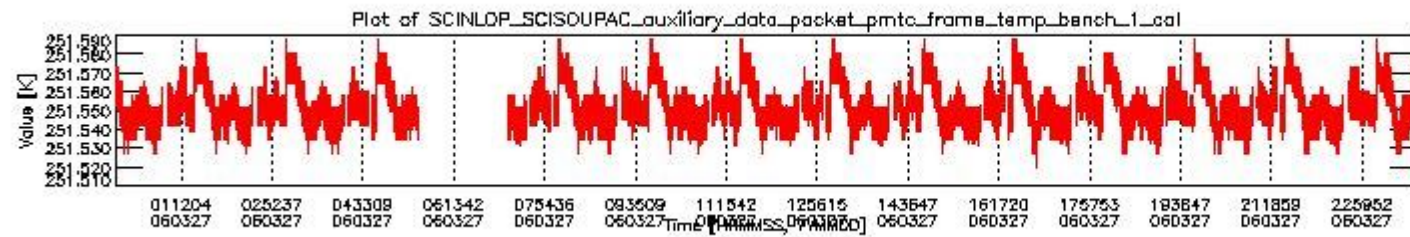
sciamachy_daily_report_level0_PFHS_5_36_N_20060327_0.PNG
