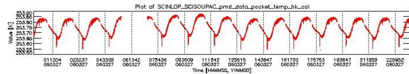
sciamachy_daily_report_level0_PFHS_5_36_N_20060327_3.PNG
