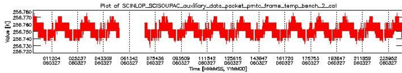
sciamachy_daily_report_level0_PFHS_5_36_N_20060327_1.PNG
