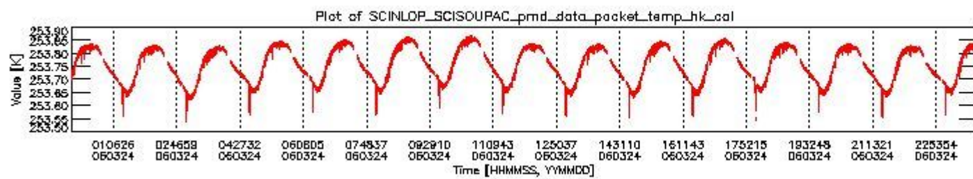
sciamachy_daily_report_level0_PFHS_5_36_N_20060324_3.PNG
