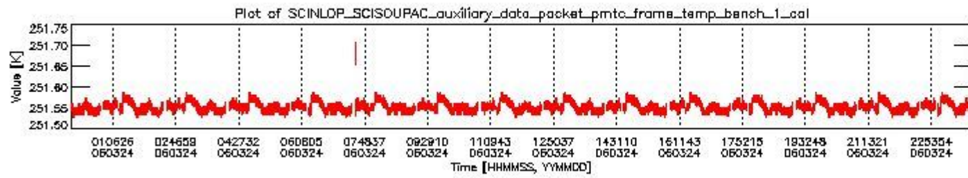
sciamachy_daily_report_level0_PFHS_5_36_N_20060324_0.PNG
