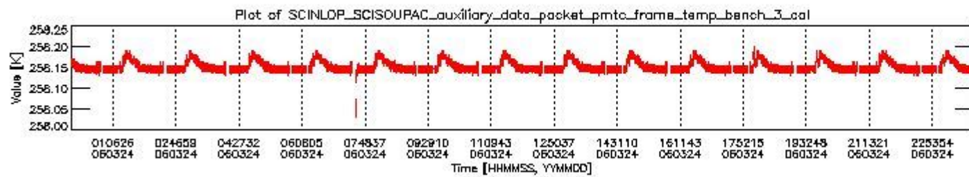
sciamachy_daily_report_level0_PFHS_5_36_N_20060324_2.PNG
