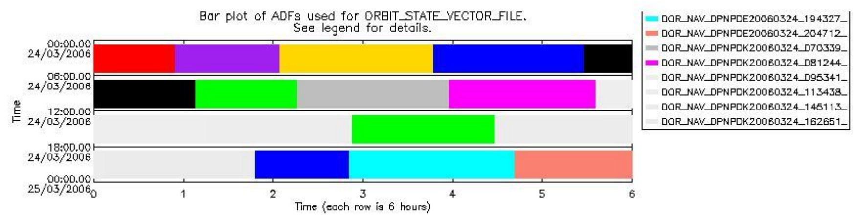
sciamachy_daily_report_level0_PFHS_5_36_N_20060324_6.PNG
