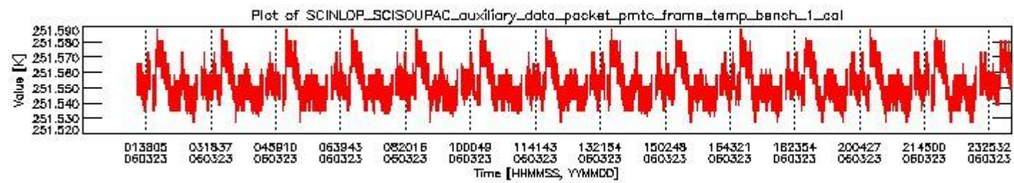
sciamachy_daily_report_level0_PFHS_5_36_N_20060323_0.PNG
