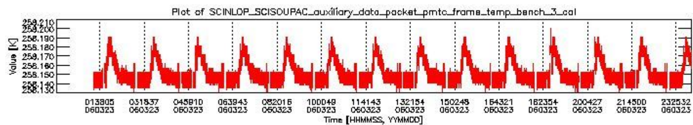
sciamachy_daily_report_level0_PFHS_5_36_N_20060323_2.PNG
