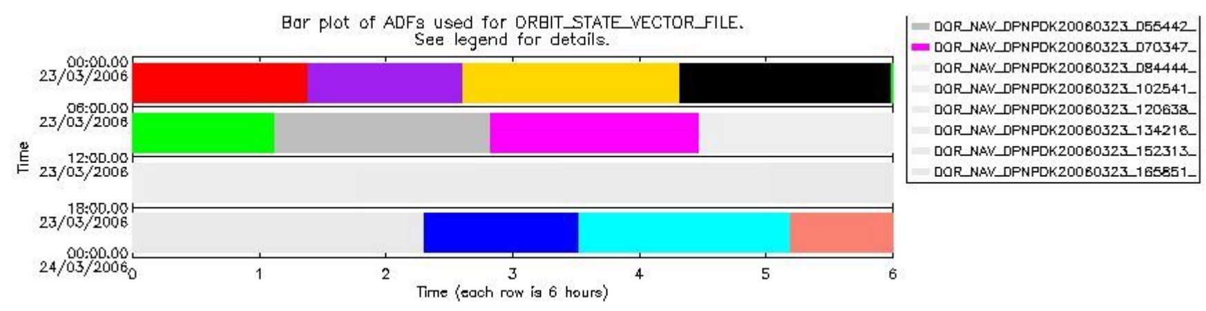
sciamachy_daily_report_level0_PFHS_5_36_N_20060323_6.PNG
