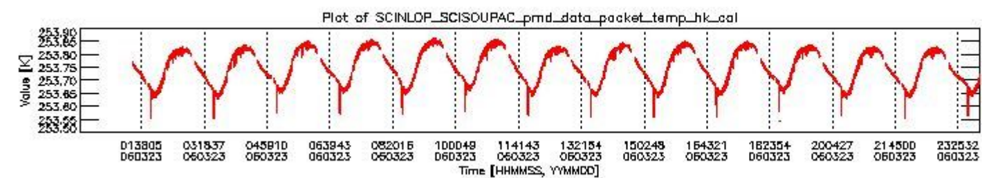
sciamachy_daily_report_level0_PFHS_5_36_N_20060323_3.PNG
