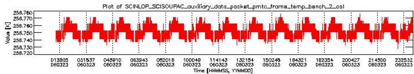
sciamachy_daily_report_level0_PFHS_5_36_N_20060323_1.PNG
