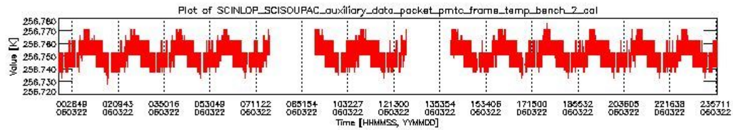
sciamachy_daily_report_level0_PFHS_5_36_N_20060322_1.PNG
