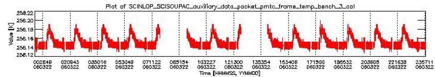
sciamachy_daily_report_level0_PFHS_5_36_N_20060322_2.PNG
