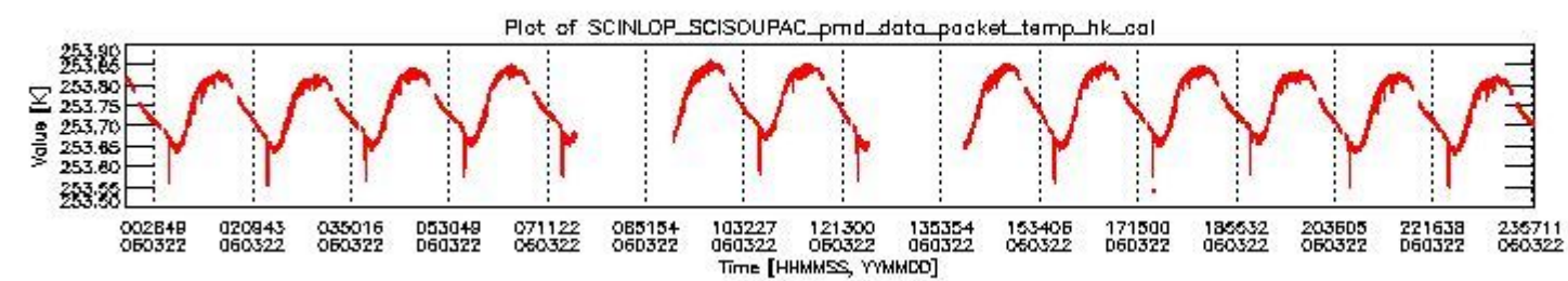
sciamachy_daily_report_level0_PFHS_5_36_N_20060322_3.PNG
