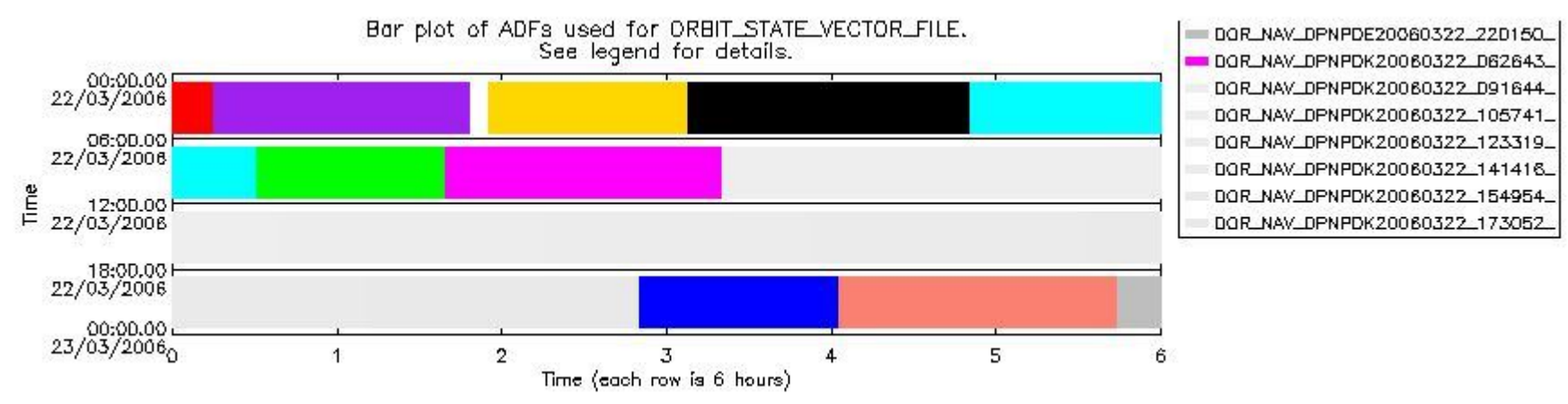
sciamachy_daily_report_level0_PFHS_5_36_N_20060322_6.PNG
