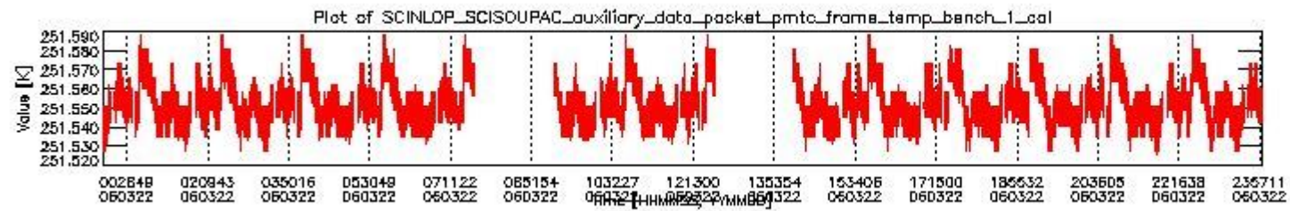
sciamachy_daily_report_level0_PFHS_5_36_N_20060322_0.PNG
