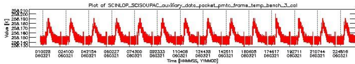
sciamachy_daily_report_level0_PFHS_5_36_N_20060321_2.PNG
