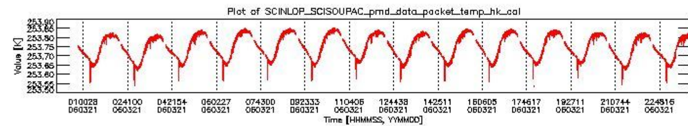
sciamachy_daily_report_level0_PFHS_5_36_N_20060321_3.PNG
