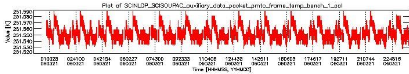
sciamachy_daily_report_level0_PFHS_5_36_N_20060321_0.PNG
