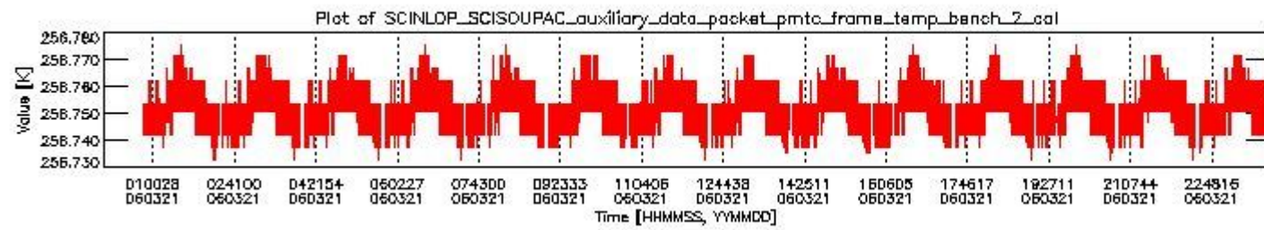
sciamachy_daily_report_level0_PFHS_5_36_N_20060321_1.PNG
