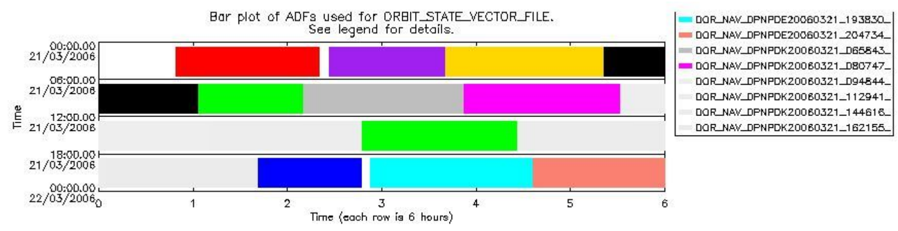
sciamachy_daily_report_level0_PFHS_5_36_N_20060321_6.PNG
