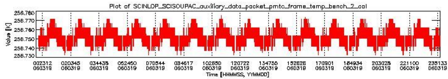
sciamachy_daily_report_level0_PFHS_5_36_N_20060319_1.PNG
