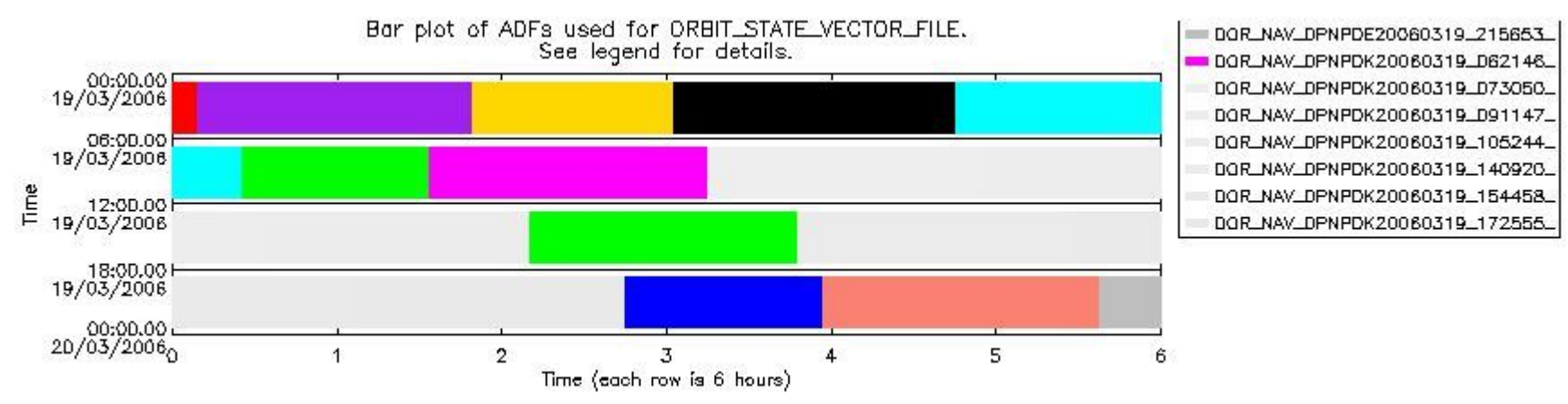
sciamachy_daily_report_level0_PFHS_5_36_N_20060319_6.PNG
