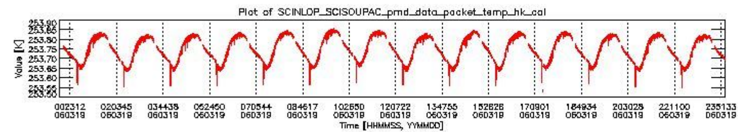
sciamachy_daily_report_level0_PFHS_5_36_N_20060319_3.PNG
