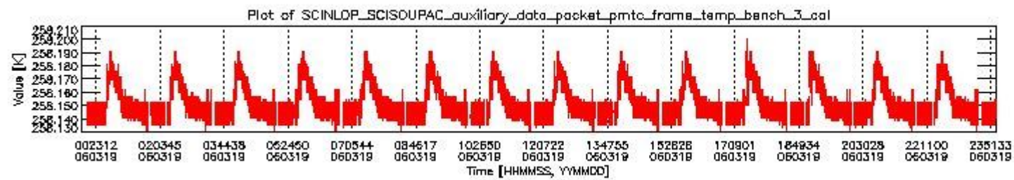
sciamachy_daily_report_level0_PFHS_5_36_N_20060319_2.PNG
