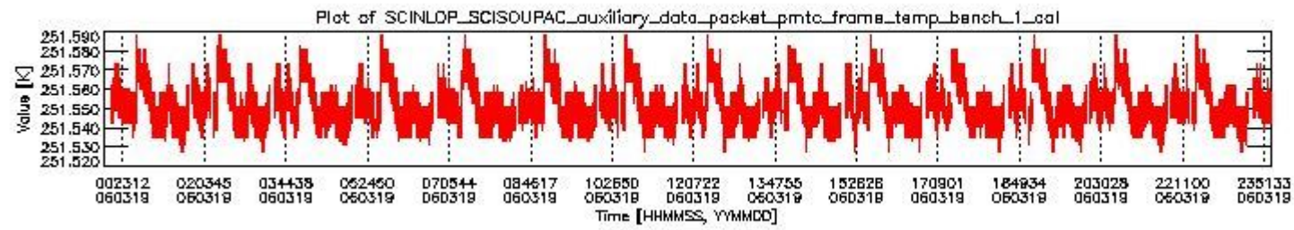
sciamachy_daily_report_level0_PFHS_5_36_N_20060319_0.PNG
