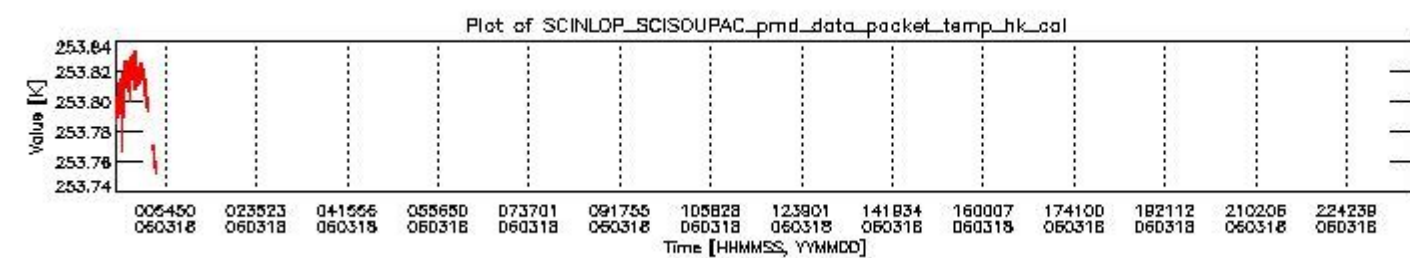
sciamachy_daily_report_level0_PFHS_5_36_N_20060318_3.PNG
