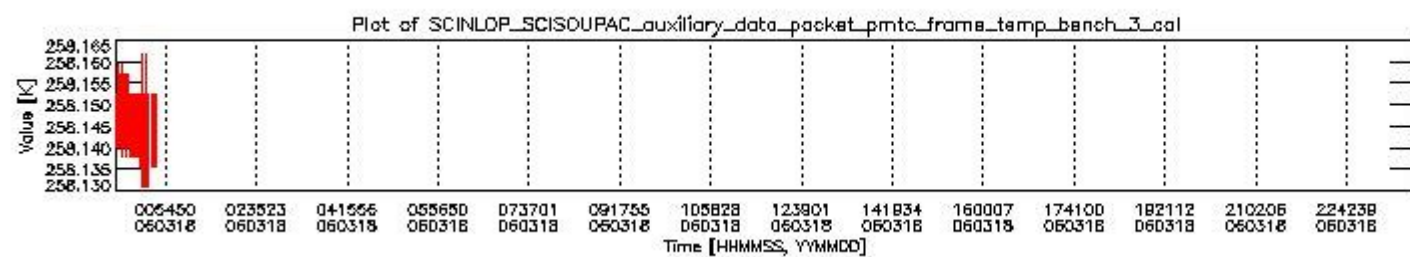
sciamachy_daily_report_level0_PFHS_5_36_N_20060318_2.PNG
