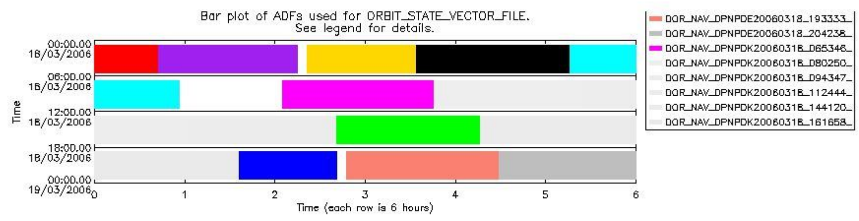
sciamachy_daily_report_level0_PFHS_5_36_N_20060318_6.PNG
