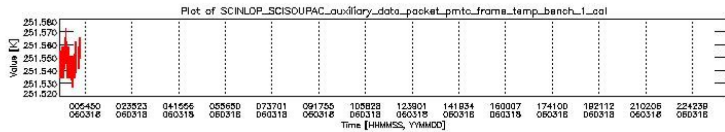
sciamachy_daily_report_level0_PFHS_5_36_N_20060318_0.PNG
