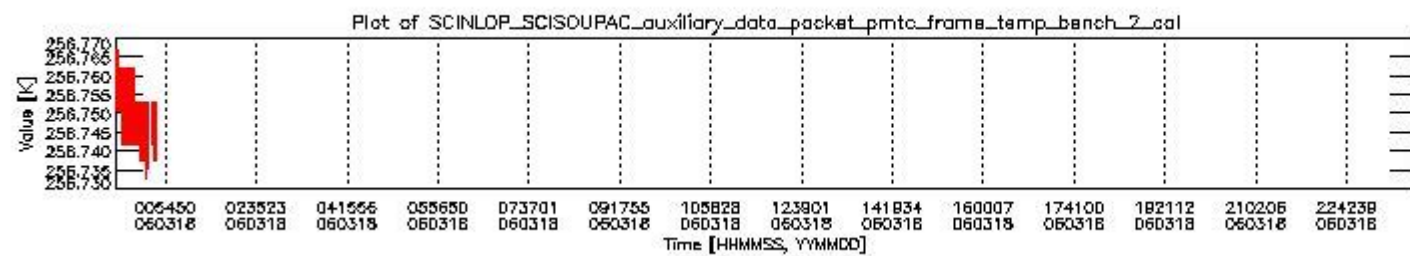
sciamachy_daily_report_level0_PFHS_5_36_N_20060318_1.PNG
