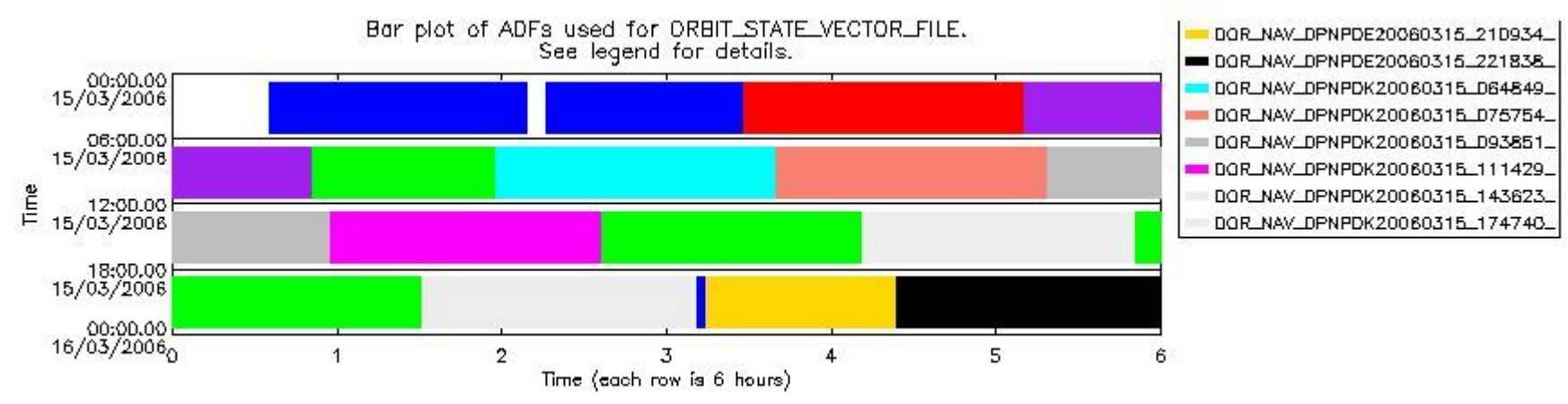
sciamachy_daily_report_level0_PFHS_5_36_N_20060315_6.PNG
