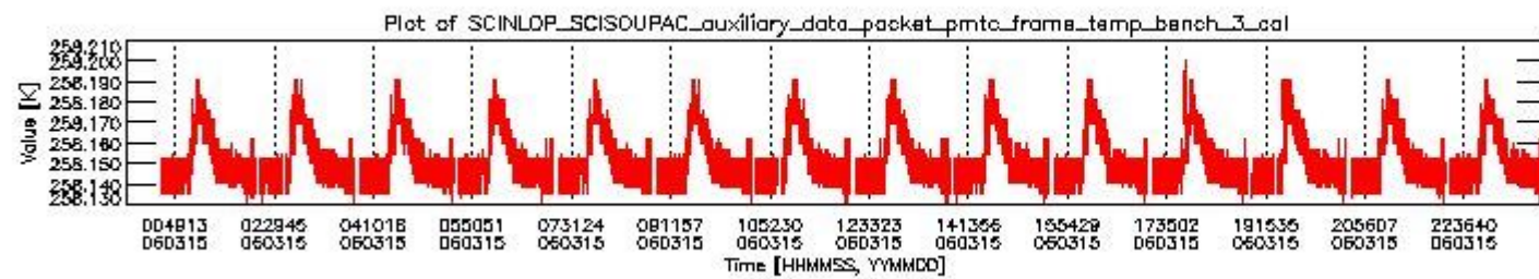
sciamachy_daily_report_level0_PFHS_5_36_N_20060315_2.PNG
