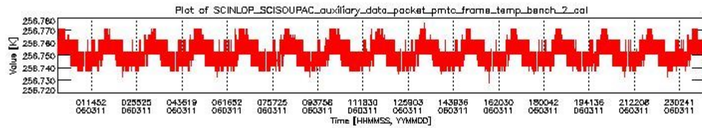
sciamachy_daily_report_level0_PFHS_5_36_N_20060311_1.PNG
