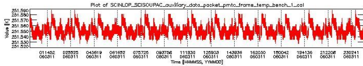
sciamachy_daily_report_level0_PFHS_5_36_N_20060311_0.PNG
