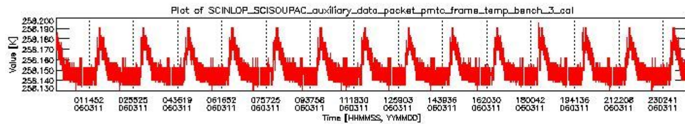
sciamachy_daily_report_level0_PFHS_5_36_N_20060311_2.PNG
