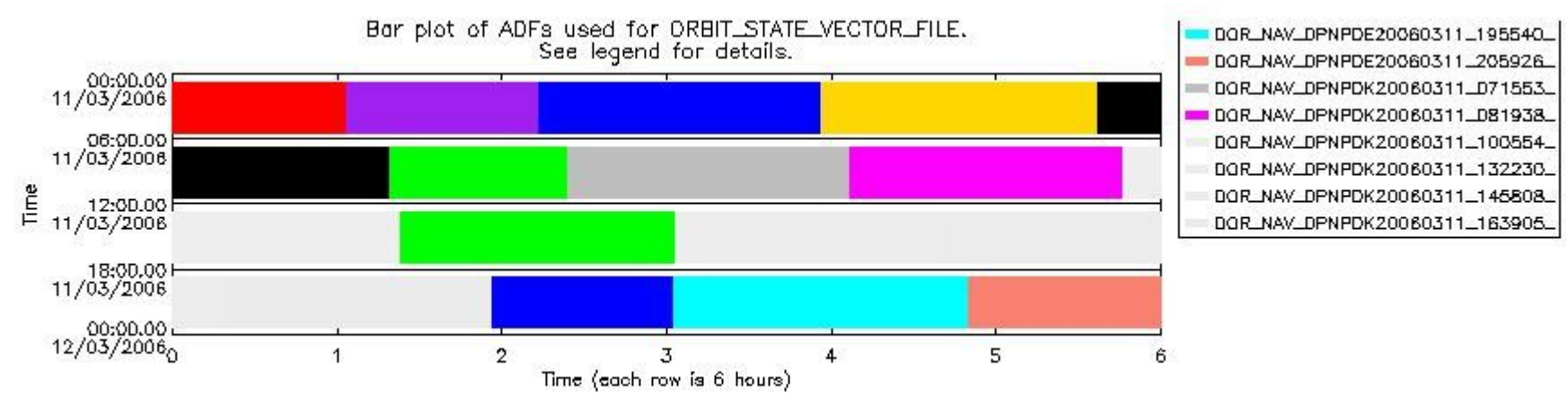
sciamachy_daily_report_level0_PFHS_5_36_N_20060311_6.PNG
