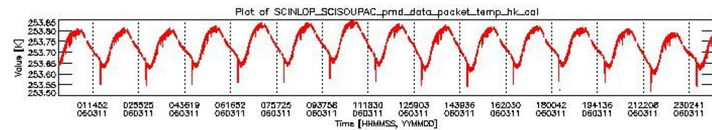
sciamachy_daily_report_level0_PFHS_5_36_N_20060311_3.PNG
