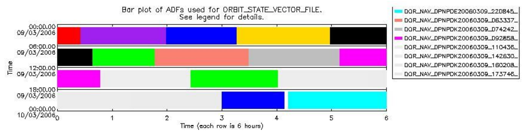
sciamachy_daily_report_level0_PFHS_5_36_N_20060309_6.PNG
