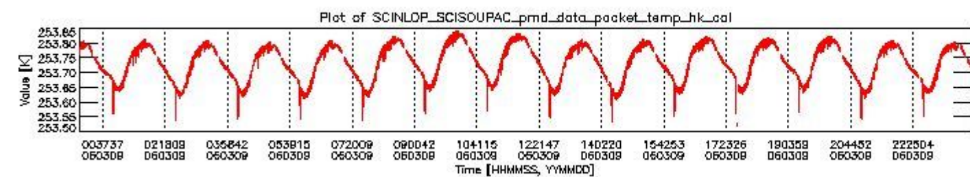
sciamachy_daily_report_level0_PFHS_5_36_N_20060309_3.PNG
