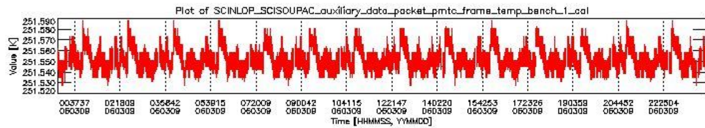
sciamachy_daily_report_level0_PFHS_5_36_N_20060309_0.PNG
