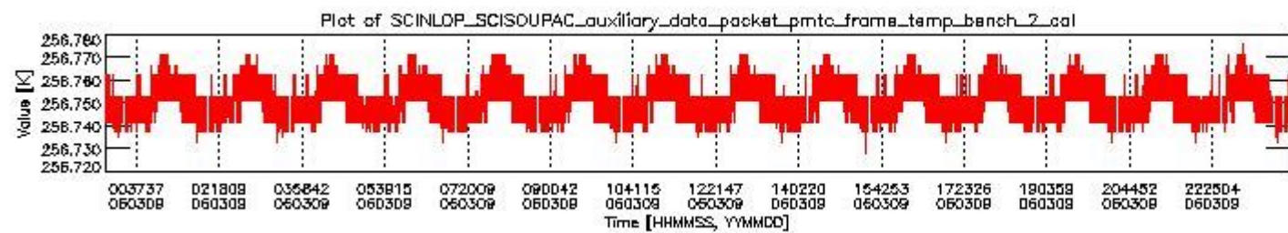
sciamachy_daily_report_level0_PFHS_5_36_N_20060309_1.PNG
