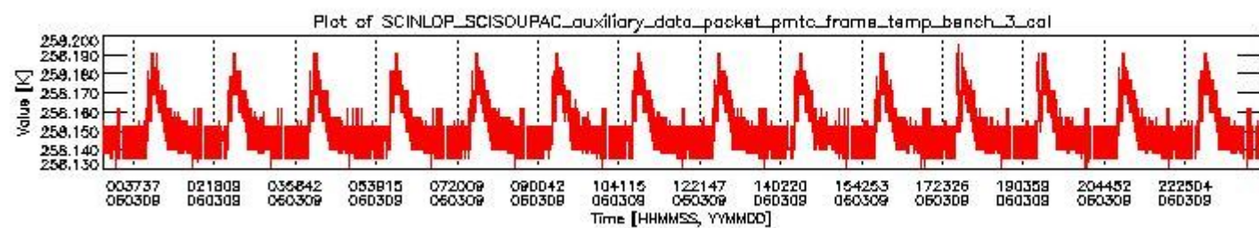
sciamachy_daily_report_level0_PFHS_5_36_N_20060309_2.PNG
