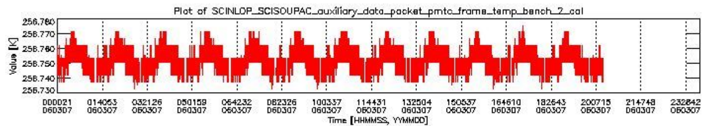
sciamachy_daily_report_level0_PFHS_5_35_N_20060307_1.PNG
