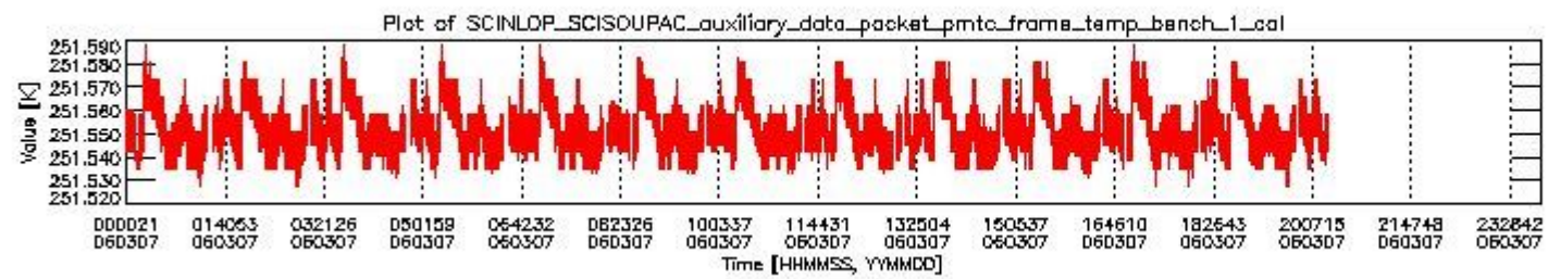
sciamachy_daily_report_level0_PFHS_5_35_N_20060307_0.PNG
