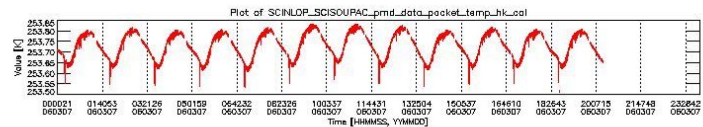
sciamachy_daily_report_level0_PFHS_5_35_N_20060307_3.PNG
