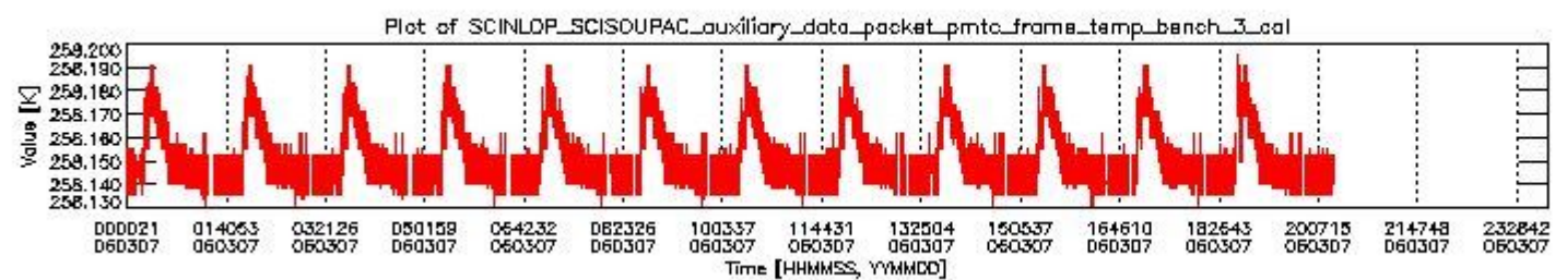
sciamachy_daily_report_level0_PFHS_5_35_N_20060307_2.PNG
