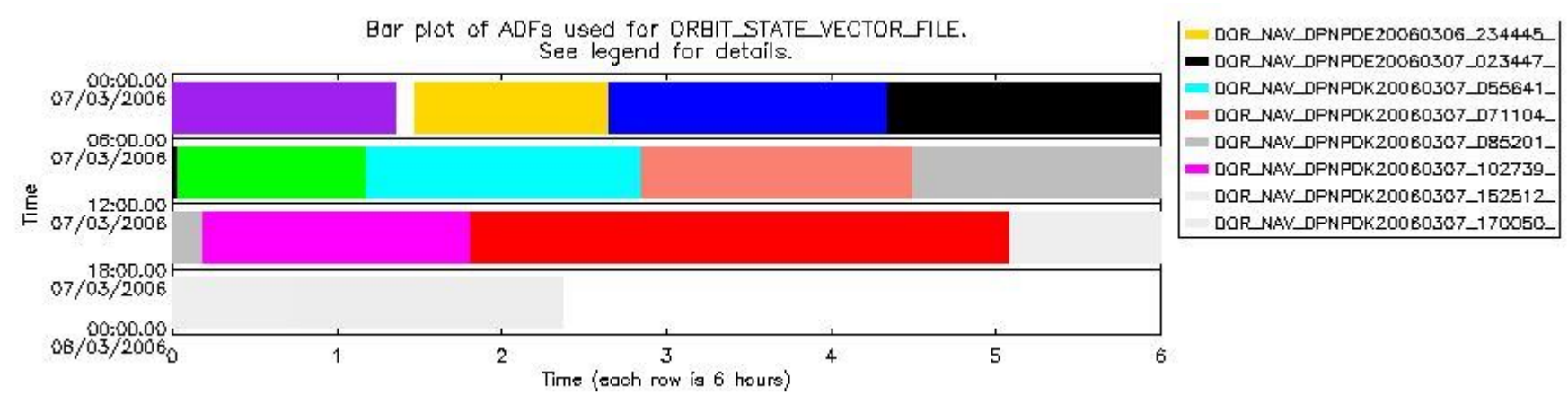
sciamachy_daily_report_level0_PFHS_5_35_N_20060307_6.PNG
