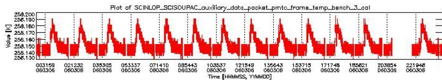
sciamachy_daily_report_level0_PFHS_5_35_N_20060306_2.PNG
