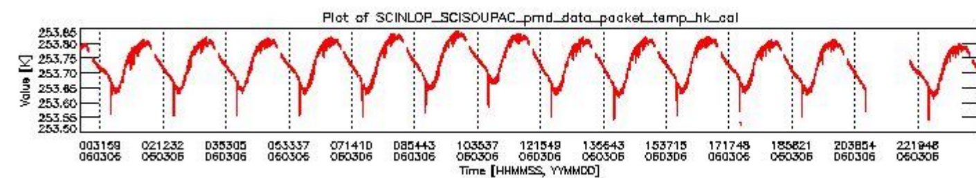
sciamachy_daily_report_level0_PFHS_5_35_N_20060306_3.PNG
