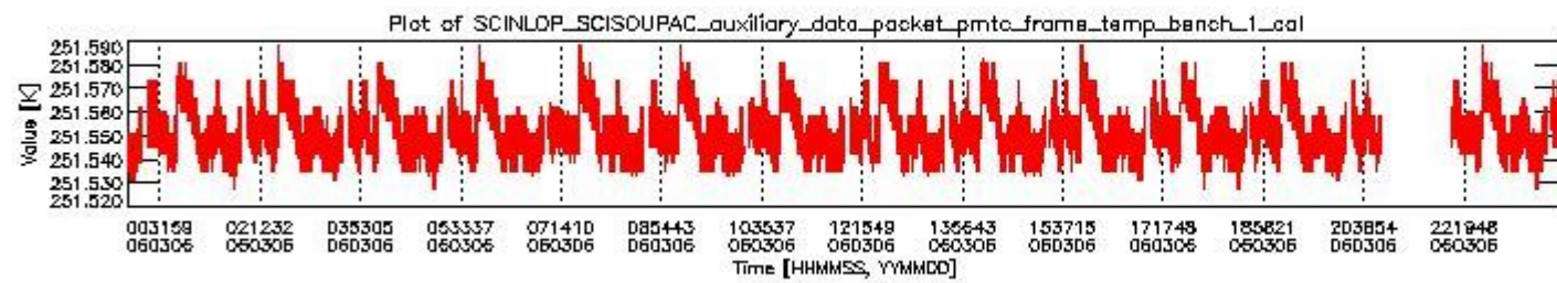
sciamachy_daily_report_level0_PFHS_5_35_N_20060306_0.PNG
