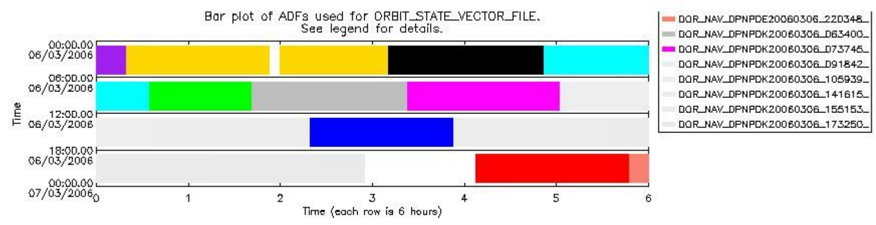
sciamachy_daily_report_level0_PFHS_5_35_N_20060306_6.PNG
