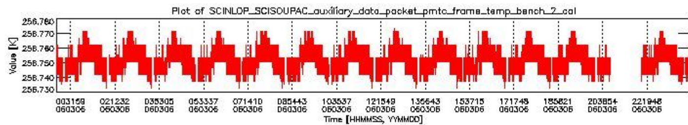
sciamachy_daily_report_level0_PFHS_5_35_N_20060306_1.PNG
