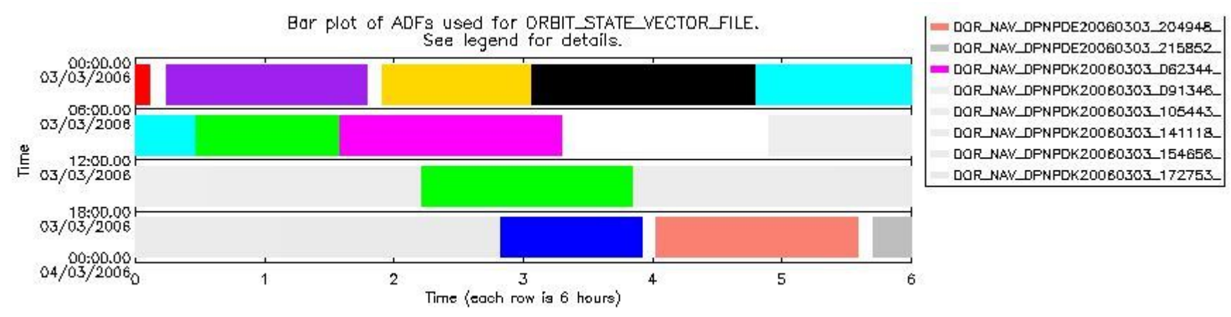
sciamachy_daily_report_level0_PFHS_5_35_N_20060303_6.PNG
