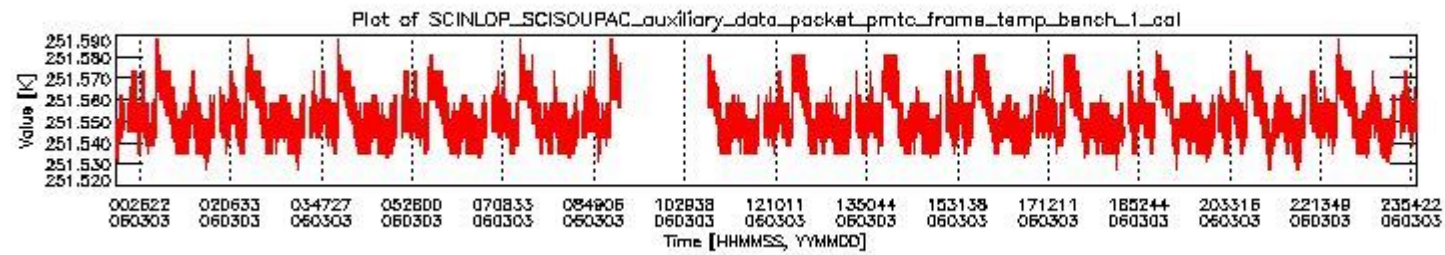
sciamachy_daily_report_level0_PFHS_5_35_N_20060303_0.PNG
