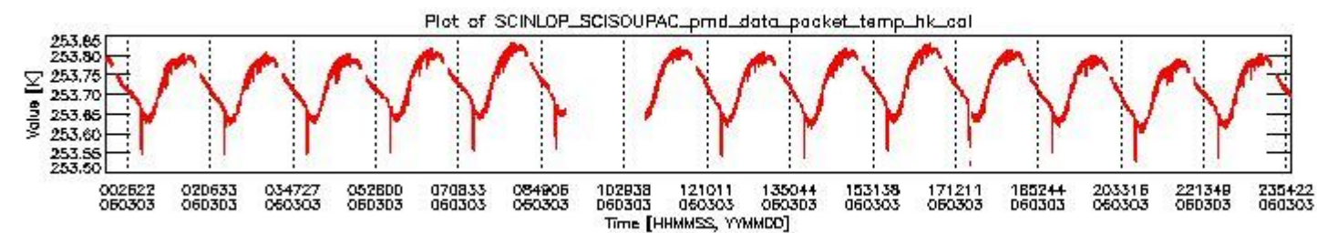
sciamachy_daily_report_level0_PFHS_5_35_N_20060303_3.PNG
