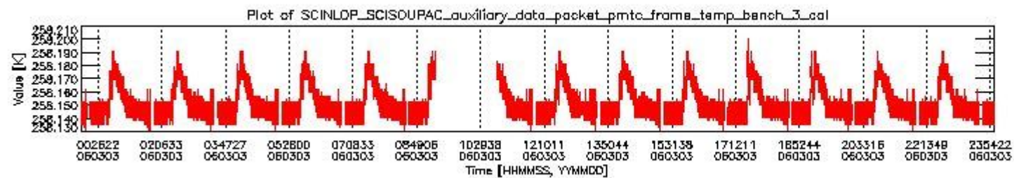
sciamachy_daily_report_level0_PFHS_5_35_N_20060303_2.PNG
