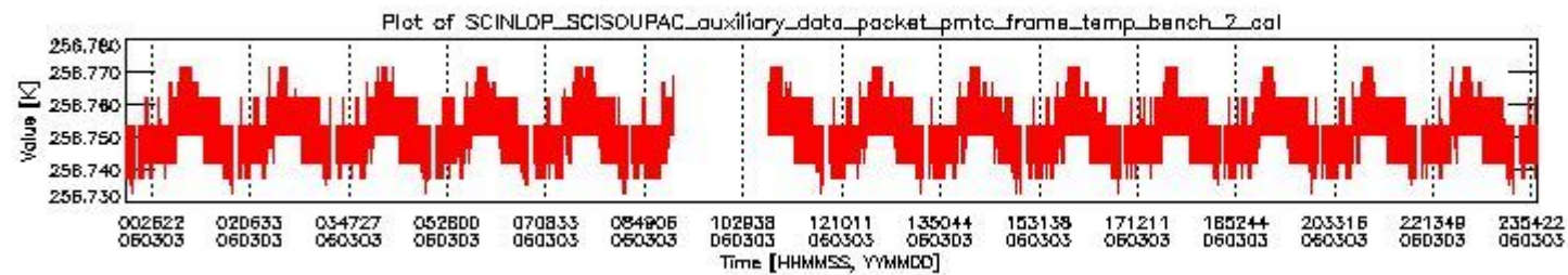
sciamachy_daily_report_level0_PFHS_5_35_N_20060303_1.PNG
