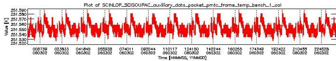
sciamachy_daily_report_level0_PFHS_5_35_N_20060302_0.PNG
