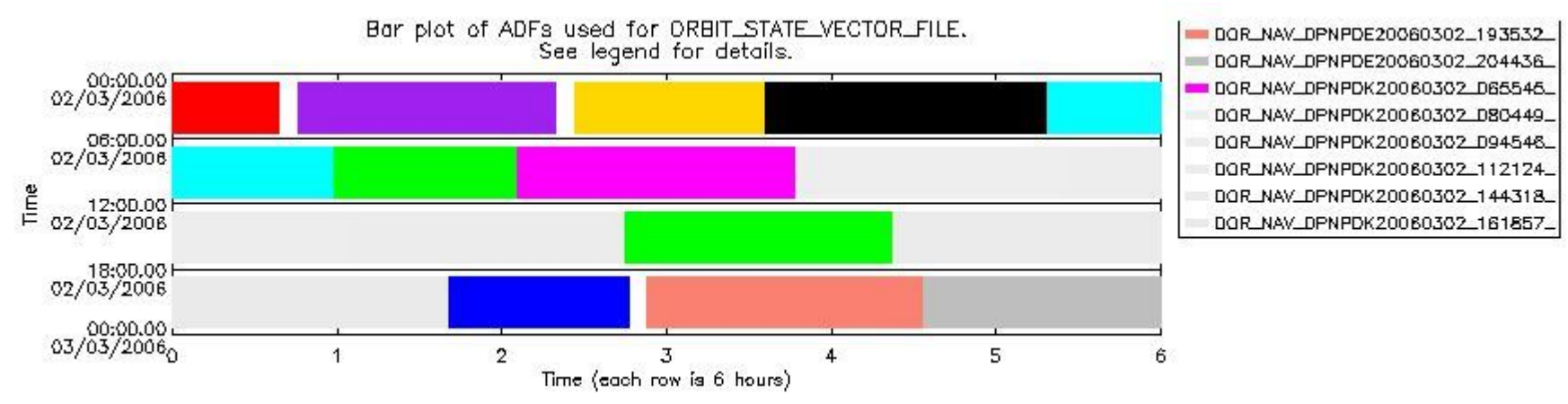
sciamachy_daily_report_level0_PFHS_5_35_N_20060302_6.PNG
