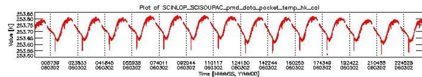
sciamachy_daily_report_level0_PFHS_5_35_N_20060302_3.PNG
