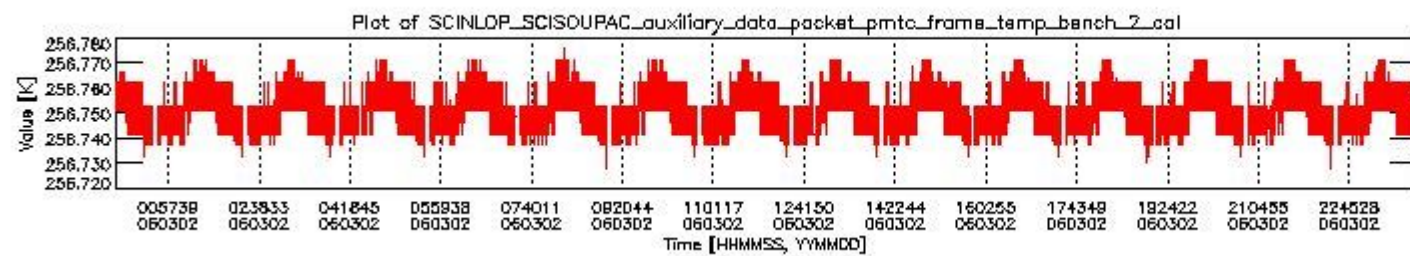
sciamachy_daily_report_level0_PFHS_5_35_N_20060302_1.PNG
