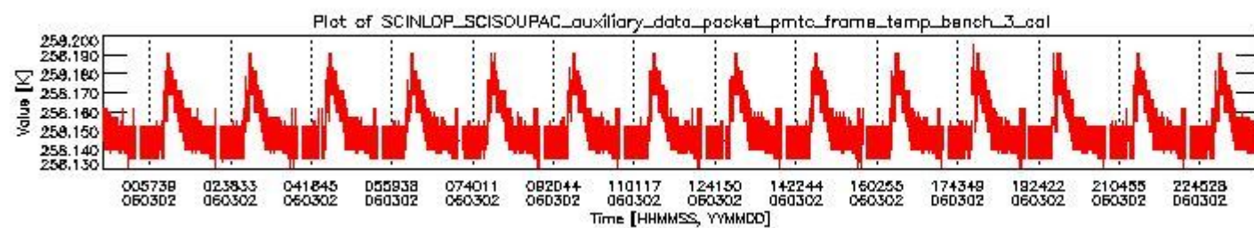
sciamachy_daily_report_level0_PFHS_5_35_N_20060302_2.PNG
