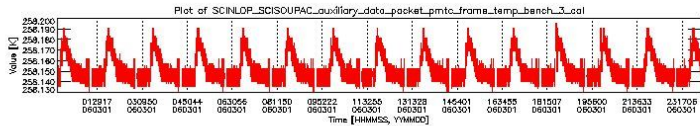
sciamachy_daily_report_level0_PFHS_5_35_N_20060301_2.PNG
