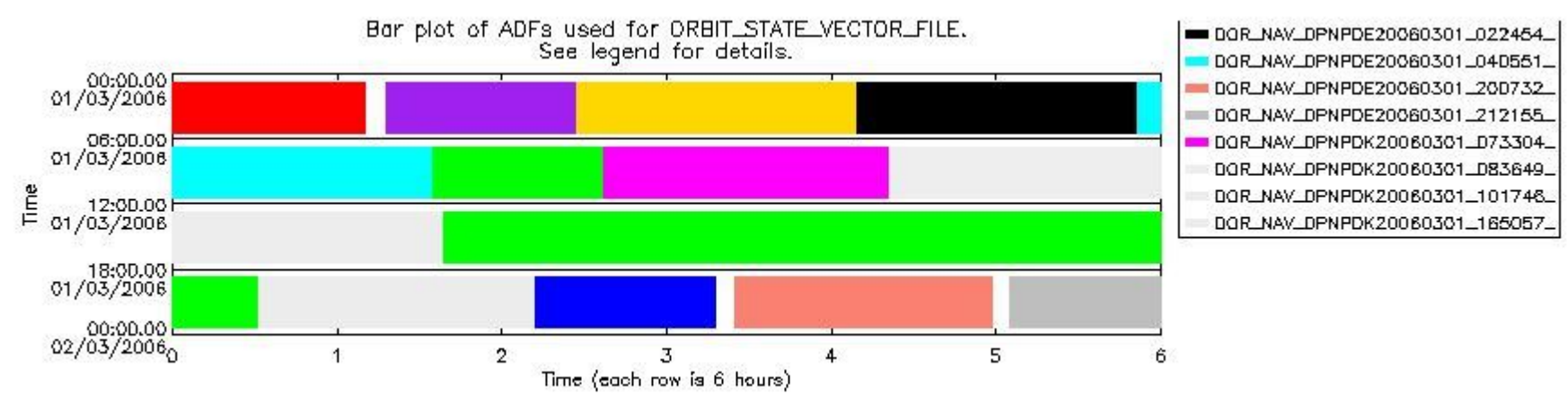
sciamachy_daily_report_level0_PFHS_5_35_N_20060301_6.PNG
