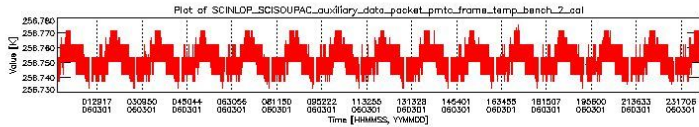
sciamachy_daily_report_level0_PFHS_5_35_N_20060301_1.PNG
