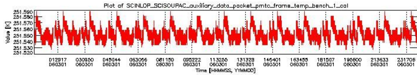
sciamachy_daily_report_level0_PFHS_5_35_N_20060301_0.PNG
