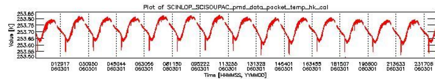
sciamachy_daily_report_level0_PFHS_5_35_N_20060301_3.PNG
