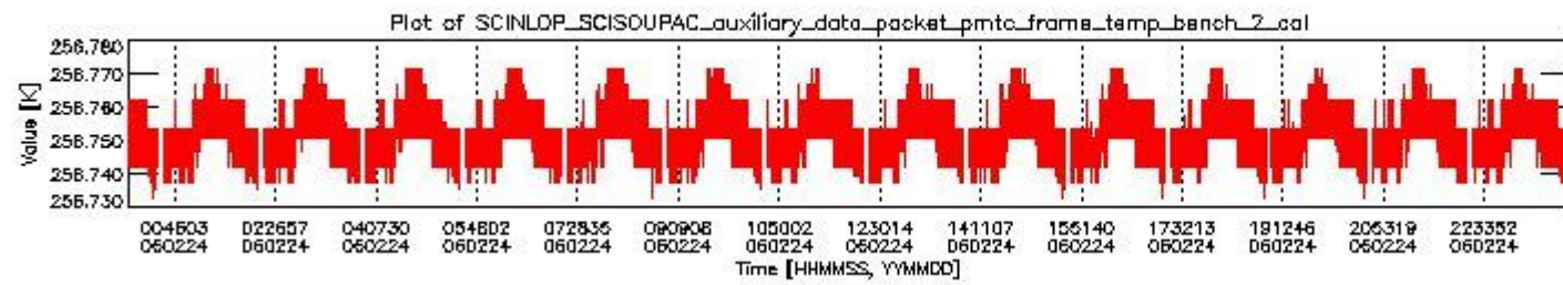
sciamachy_daily_report_level0_PFHS_5_35_N_20060224_1.PNG
