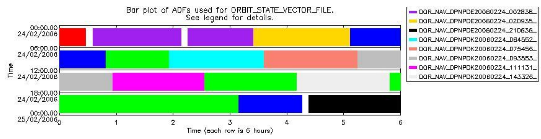
sciamachy_daily_report_level0_PFHS_5_35_N_20060224_6.PNG
