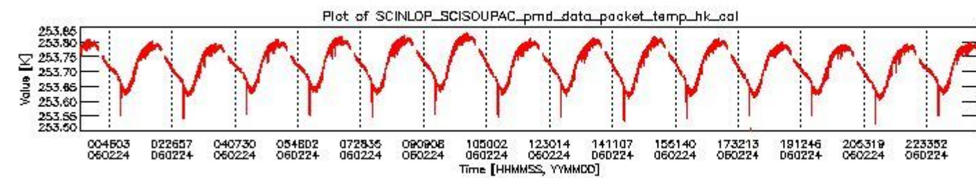
sciamachy_daily_report_level0_PFHS_5_35_N_20060224_3.PNG
