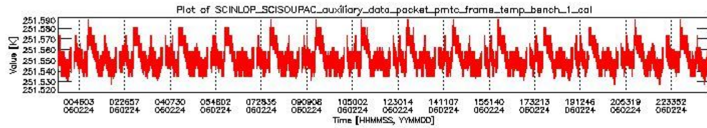
sciamachy_daily_report_level0_PFHS_5_35_N_20060224_0.PNG
