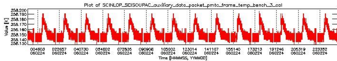
sciamachy_daily_report_level0_PFHS_5_35_N_20060224_2.PNG
