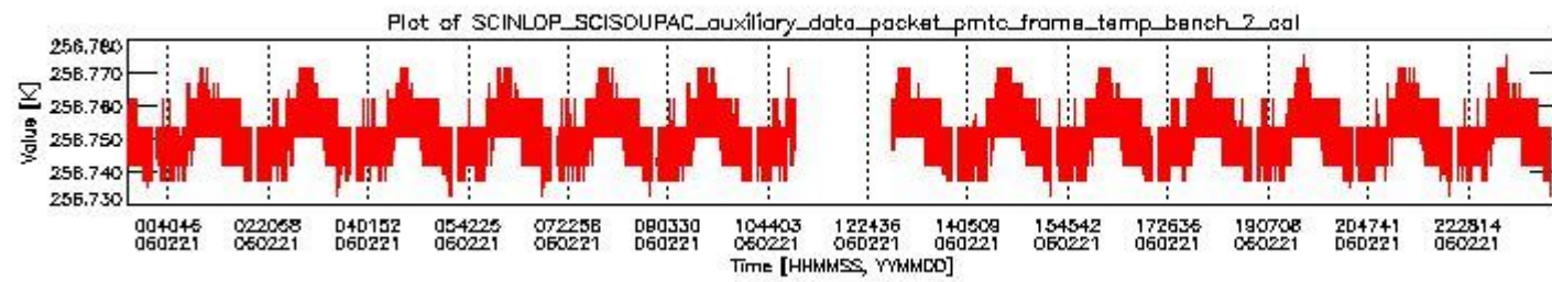
sciamachy_daily_report_level0_PFHS_5_35_N_20060221_1.PNG
