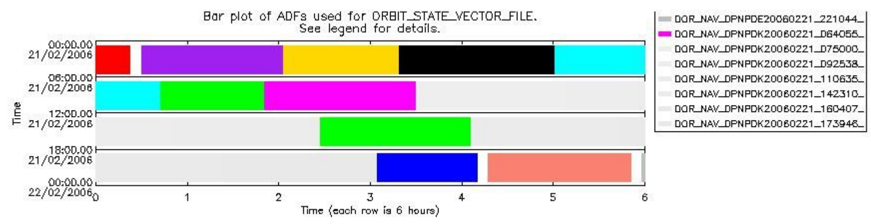
sciamachy_daily_report_level0_PFHS_5_35_N_20060221_6.PNG
