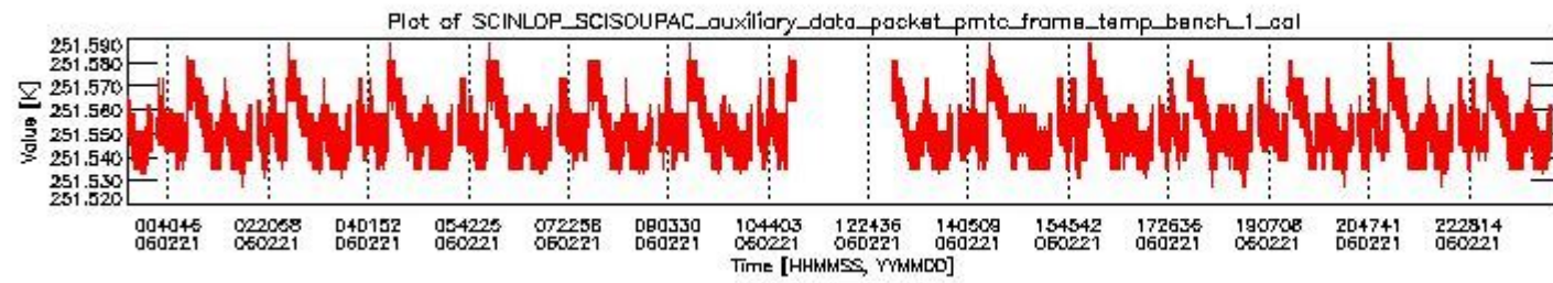
sciamachy_daily_report_level0_PFHS_5_35_N_20060221_0.PNG
