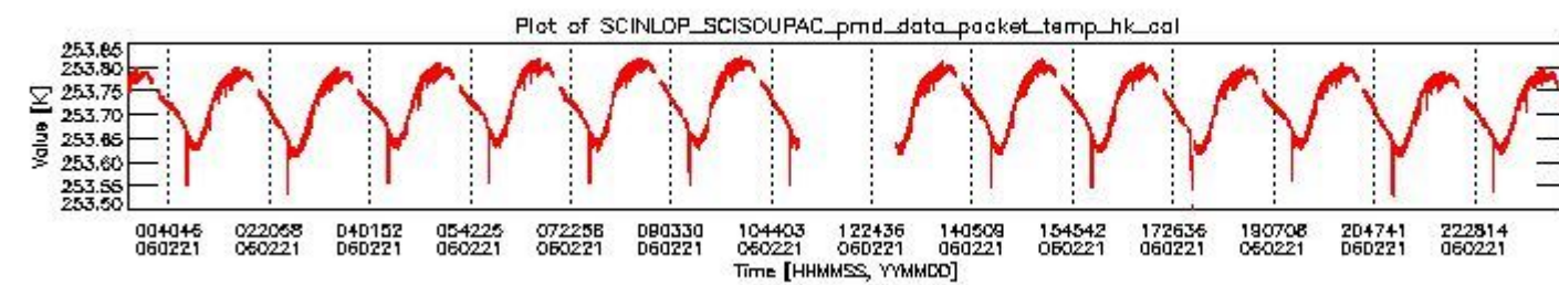
sciamachy_daily_report_level0_PFHS_5_35_N_20060221_3.PNG
