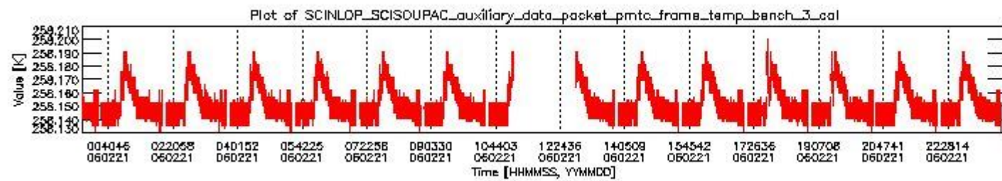
sciamachy_daily_report_level0_PFHS_5_35_N_20060221_2.PNG
