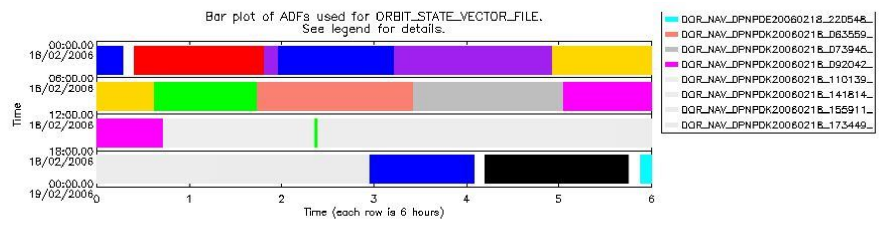
sciamachy_daily_report_level0_PFHS_5_35_N_20060218_6.PNG
