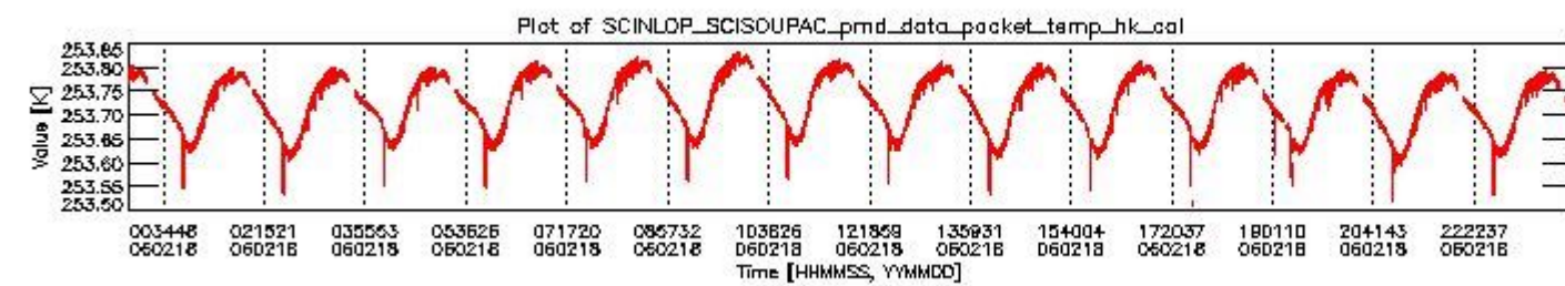
sciamachy_daily_report_level0_PFHS_5_35_N_20060218_3.PNG
