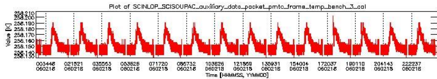
sciamachy_daily_report_level0_PFHS_5_35_N_20060218_2.PNG
