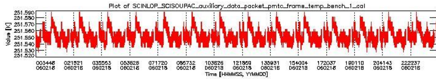
sciamachy_daily_report_level0_PFHS_5_35_N_20060218_0.PNG
