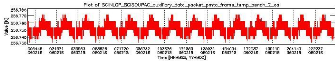
sciamachy_daily_report_level0_PFHS_5_35_N_20060218_1.PNG
