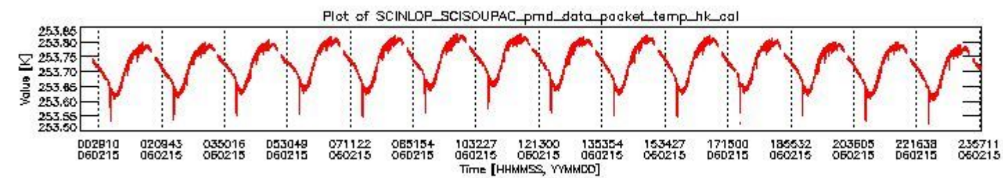
sciamachy_daily_report_level0_PFHS_5_35_N_20060215_3.PNG
