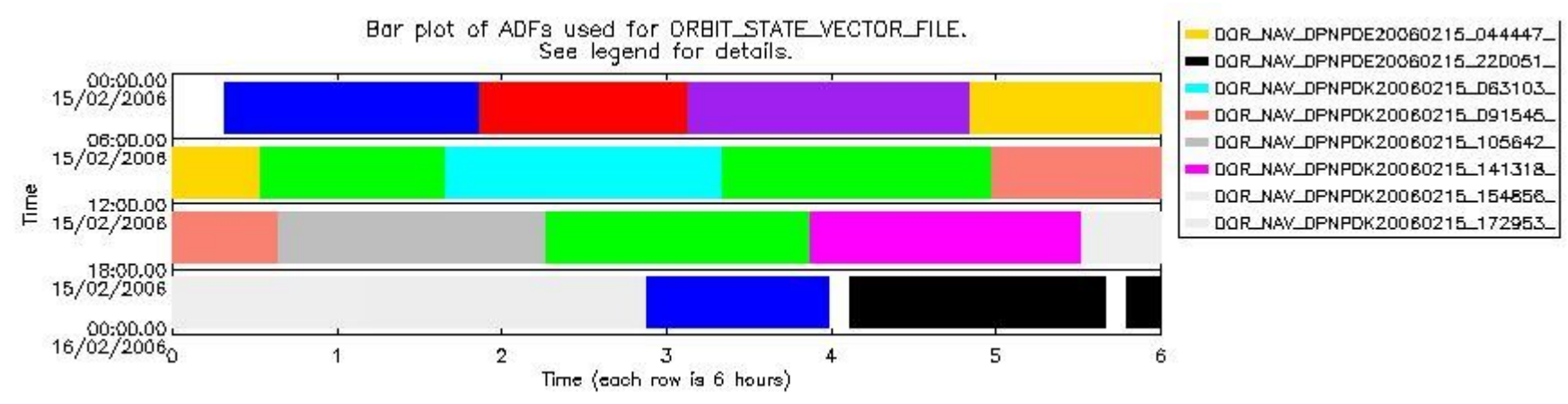
sciamachy_daily_report_level0_PFHS_5_35_N_20060215_6.PNG
