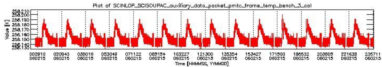
sciamachy_daily_report_level0_PFHS_5_35_N_20060215_2.PNG
