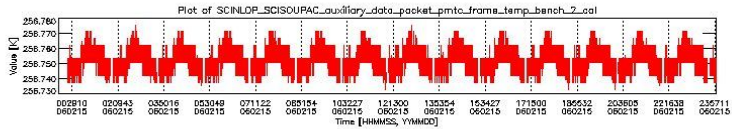
sciamachy_daily_report_level0_PFHS_5_35_N_20060215_1.PNG
