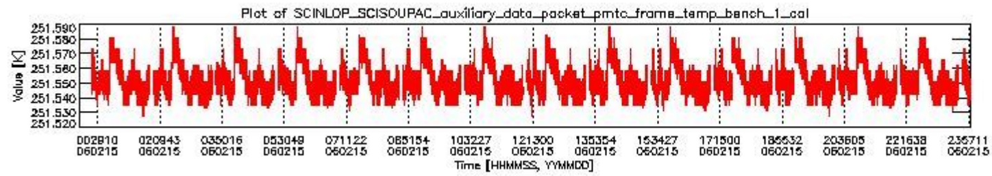
sciamachy_daily_report_level0_PFHS_5_35_N_20060215_0.PNG
