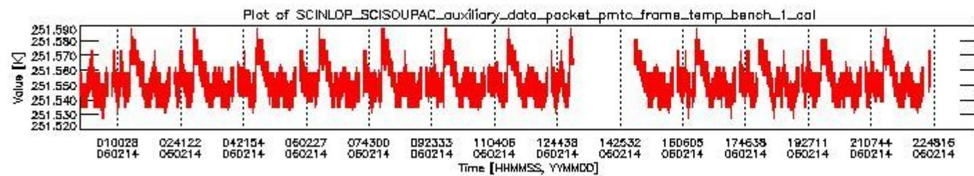
sciamachy_daily_report_level0_PFHS_5_35_N_20060214_0.PNG
