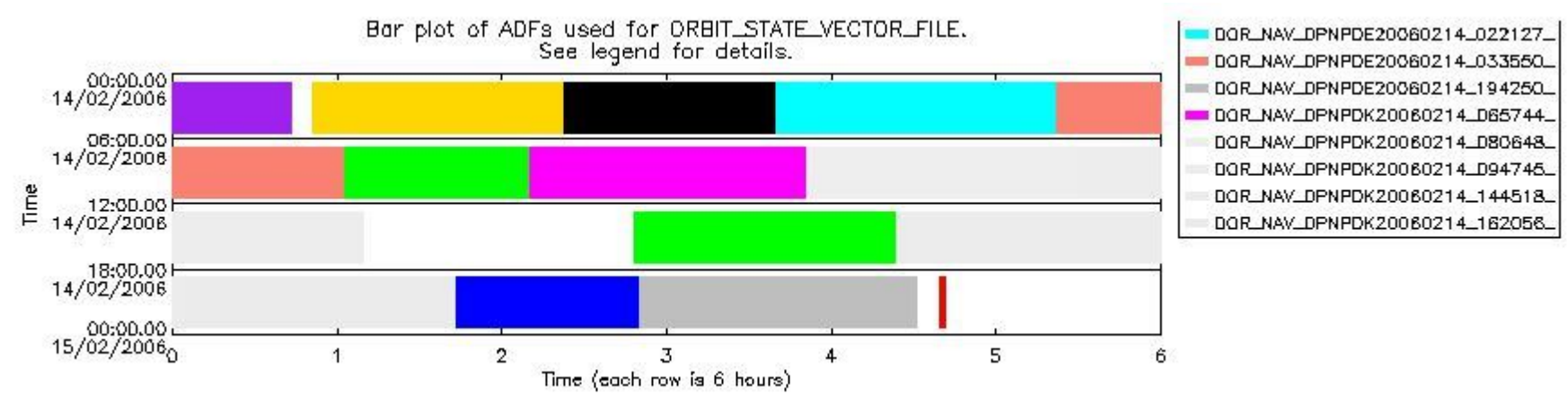
sciamachy_daily_report_level0_PFHS_5_35_N_20060214_6.PNG
