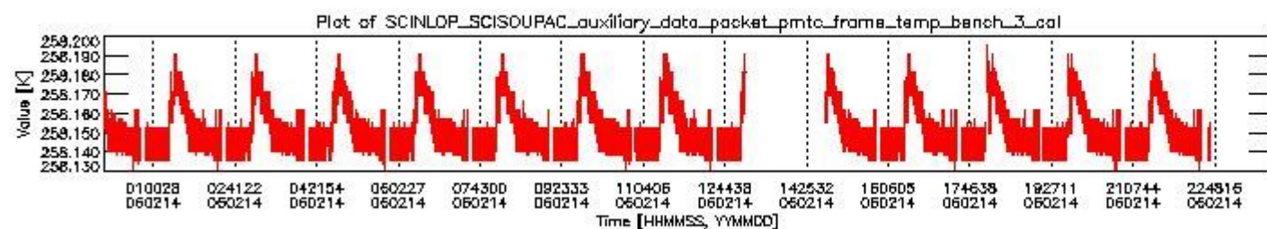
sciamachy_daily_report_level0_PFHS_5_35_N_20060214_2.PNG
