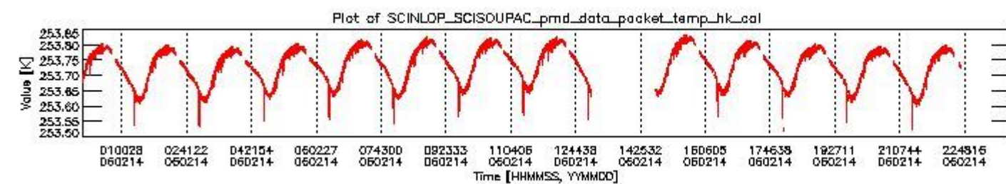
sciamachy_daily_report_level0_PFHS_5_35_N_20060214_3.PNG
