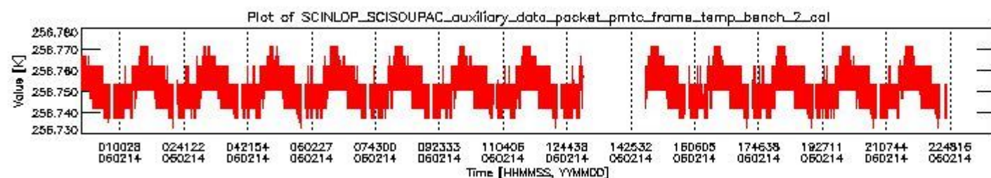
sciamachy_daily_report_level0_PFHS_5_35_N_20060214_1.PNG
