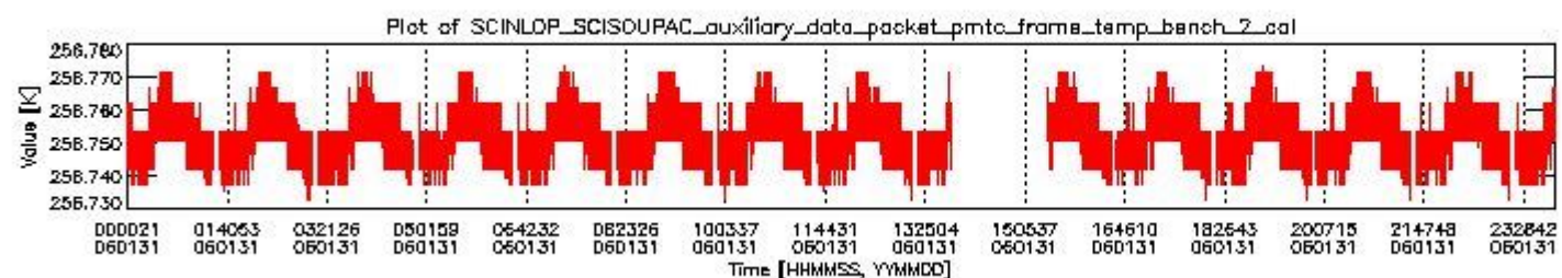
sciamachy_daily_report_level0_PFHS_5_35_N_20060131_1.PNG
