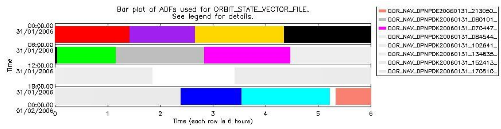
sciamachy_daily_report_level0_PFHS_5_35_N_20060131_6.PNG
