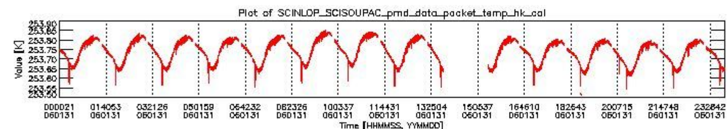
sciamachy_daily_report_level0_PFHS_5_35_N_20060131_3.PNG
