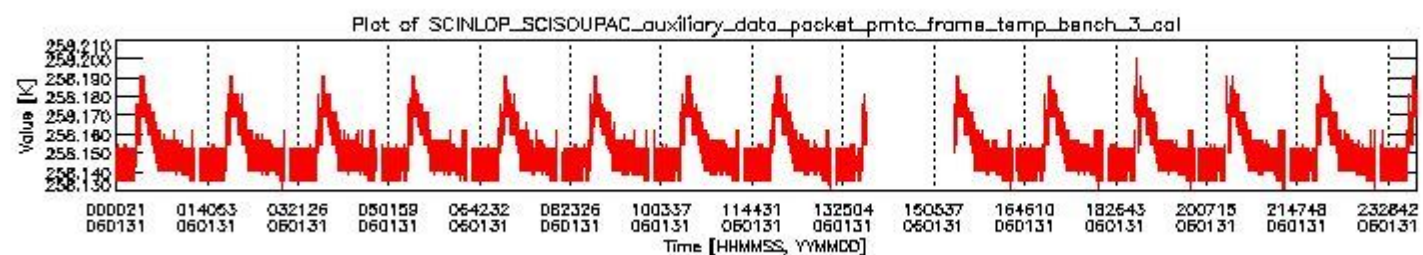
sciamachy_daily_report_level0_PFHS_5_35_N_20060131_2.PNG
