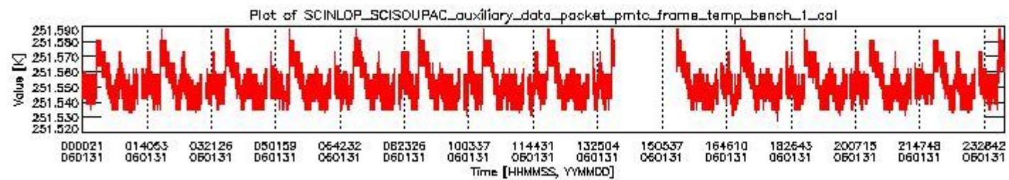
sciamachy_daily_report_level0_PFHS_5_35_N_20060131_0.PNG
