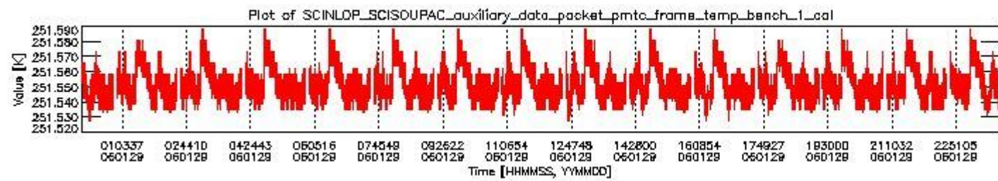
sciamachy_daily_report_level0_PFHS_5_35_N_20060129_0.PNG
