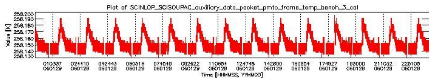
sciamachy_daily_report_level0_PFHS_5_35_N_20060129_2.PNG
