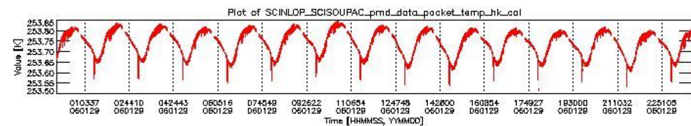
sciamachy_daily_report_level0_PFHS_5_35_N_20060129_3.PNG
