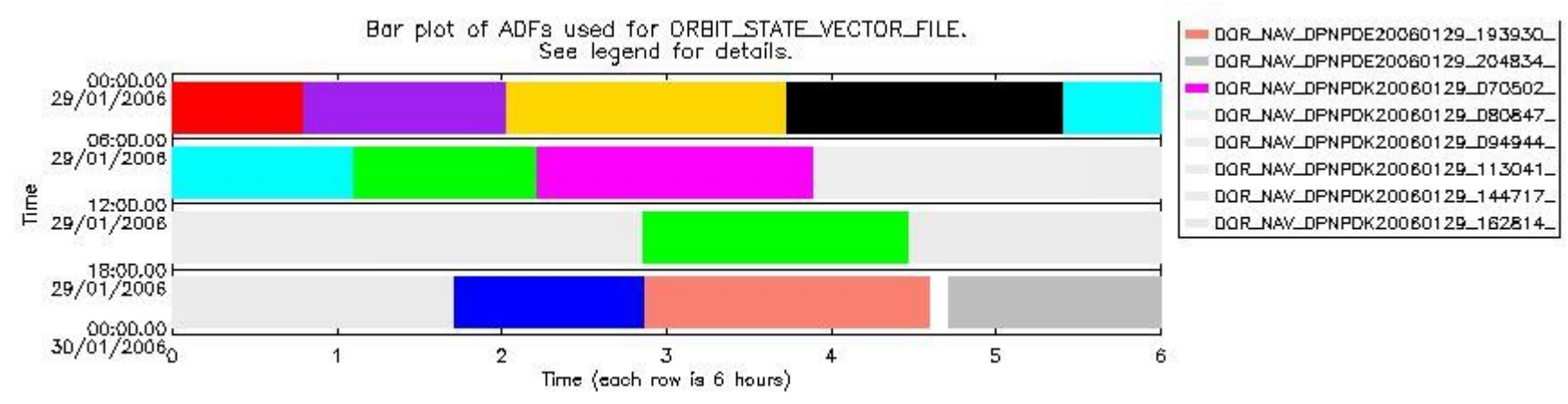
sciamachy_daily_report_level0_PFHS_5_35_N_20060129_6.PNG
