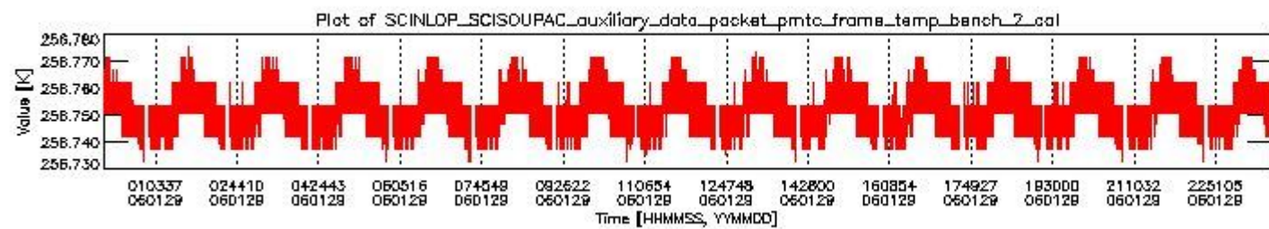
sciamachy_daily_report_level0_PFHS_5_35_N_20060129_1.PNG
