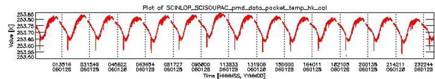
sciamachy_daily_report_level0_PFHS_5_35_N_20060128_3.PNG
