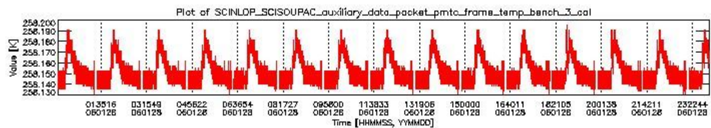
sciamachy_daily_report_level0_PFHS_5_35_N_20060128_2.PNG
