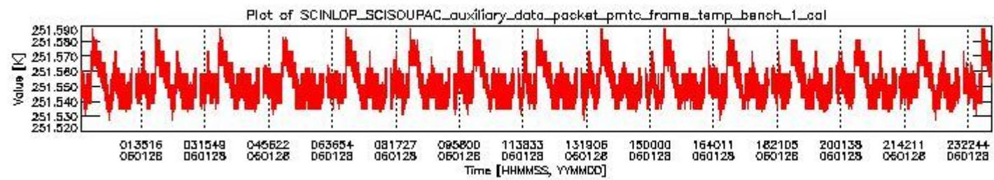
sciamachy_daily_report_level0_PFHS_5_35_N_20060128_0.PNG
