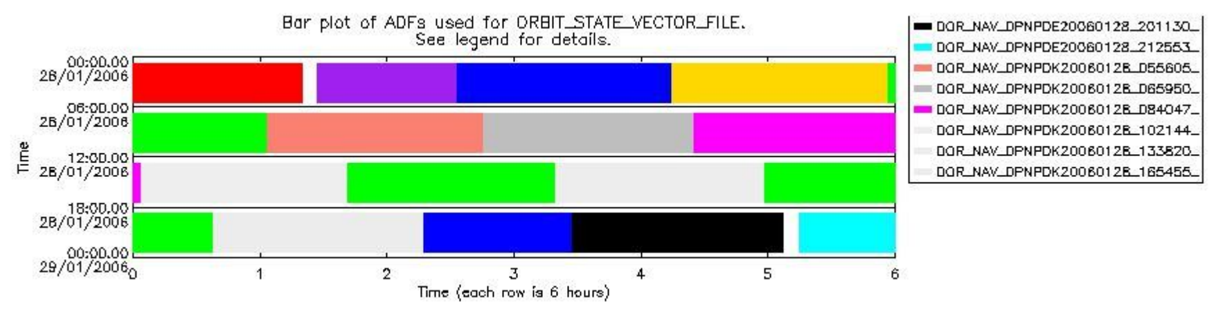
sciamachy_daily_report_level0_PFHS_5_35_N_20060128_6.PNG
