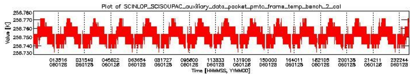
sciamachy_daily_report_level0_PFHS_5_35_N_20060128_1.PNG
