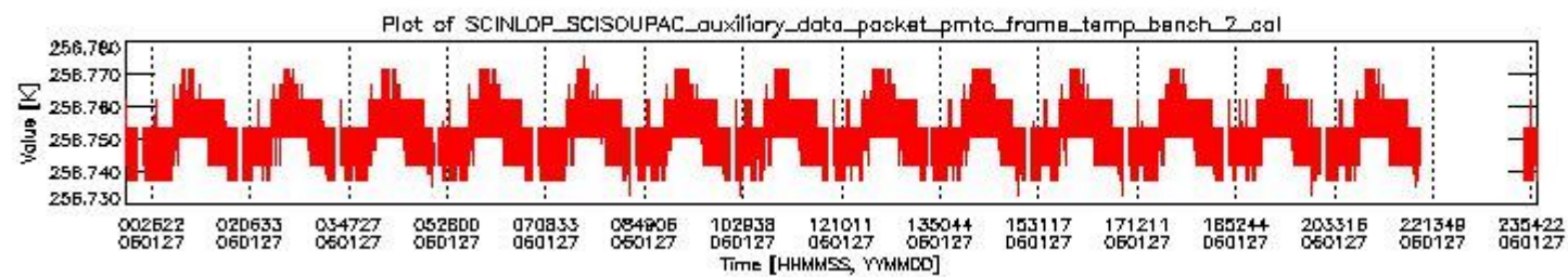
sciamachy_daily_report_level0_PFHS_5_35_N_20060127_1.PNG
