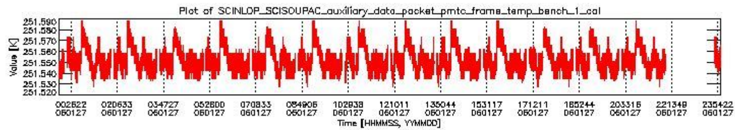
sciamachy_daily_report_level0_PFHS_5_35_N_20060127_0.PNG
