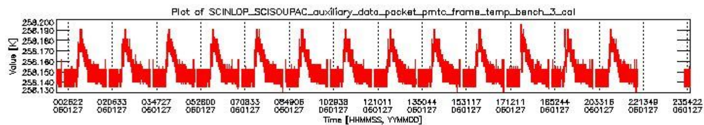
sciamachy_daily_report_level0_PFHS_5_35_N_20060127_2.PNG
