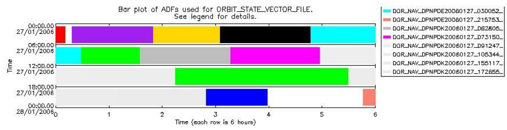
sciamachy_daily_report_level0_PFHS_5_35_N_20060127_6.PNG
