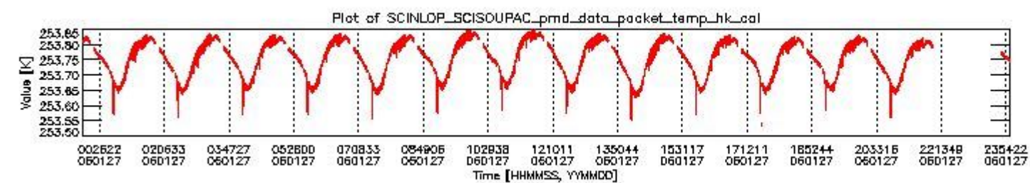
sciamachy_daily_report_level0_PFHS_5_35_N_20060127_3.PNG
