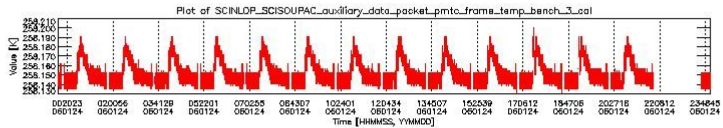
sciamachy_daily_report_level0_PFHS_5_35_N_20060124_2.PNG
