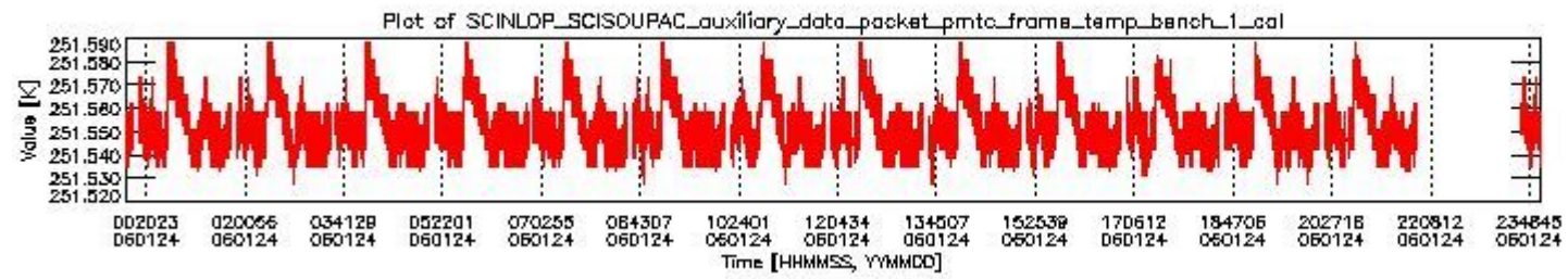
sciamachy_daily_report_level0_PFHS_5_35_N_20060124_0.PNG
