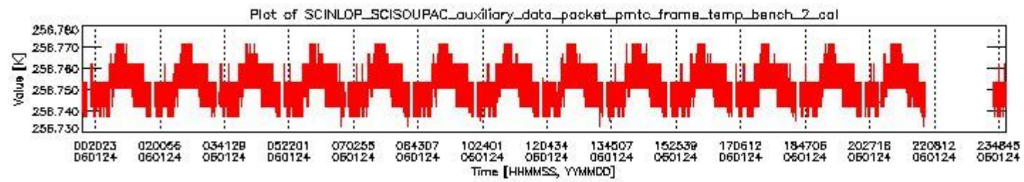
sciamachy_daily_report_level0_PFHS_5_35_N_20060124_1.PNG
