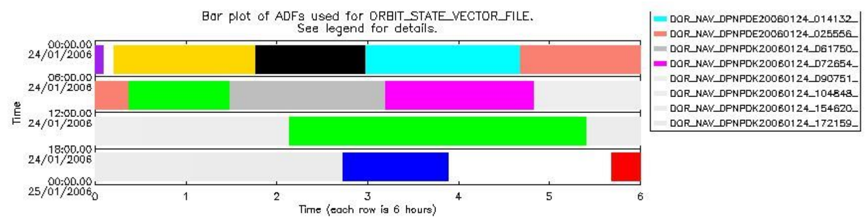
sciamachy_daily_report_level0_PFHS_5_35_N_20060124_6.PNG
