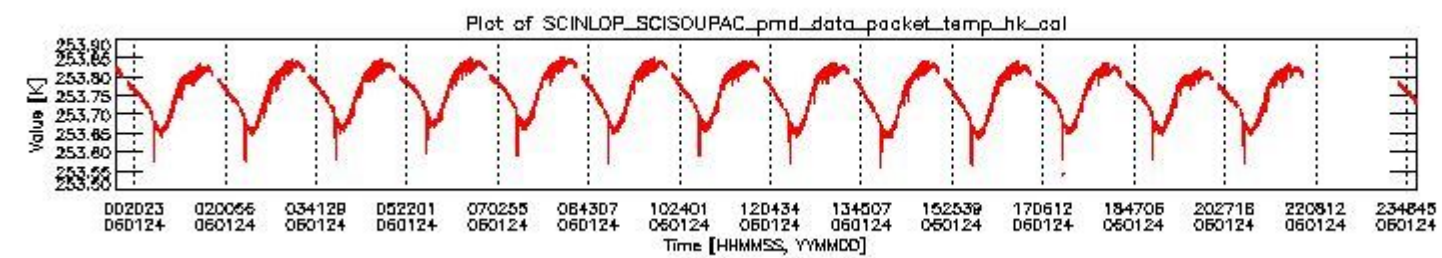
sciamachy_daily_report_level0_PFHS_5_35_N_20060124_3.PNG
