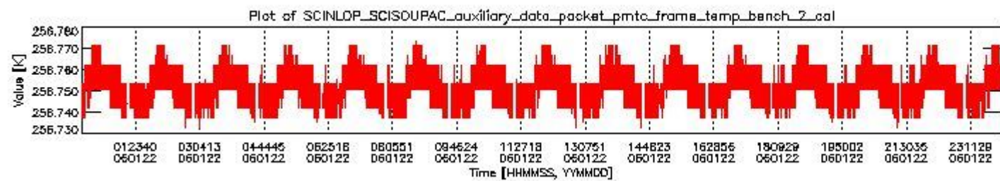
sciamachy_daily_report_level0_PFHS_5_35_N_20060122_1.PNG
