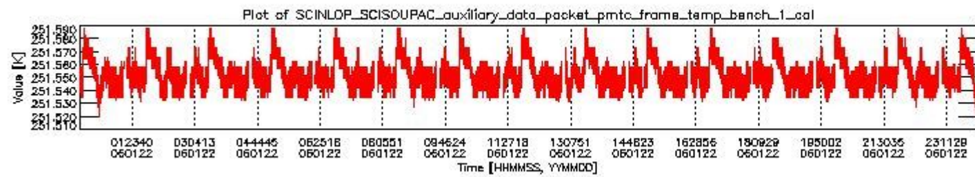
sciamachy_daily_report_level0_PFHS_5_35_N_20060122_0.PNG
