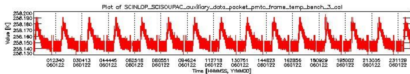
sciamachy_daily_report_level0_PFHS_5_35_N_20060122_2.PNG
