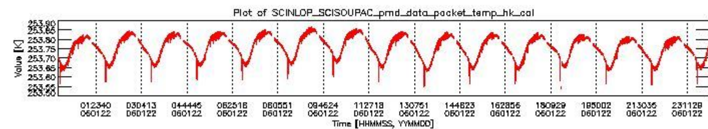
sciamachy_daily_report_level0_PFHS_5_35_N_20060122_3.PNG
