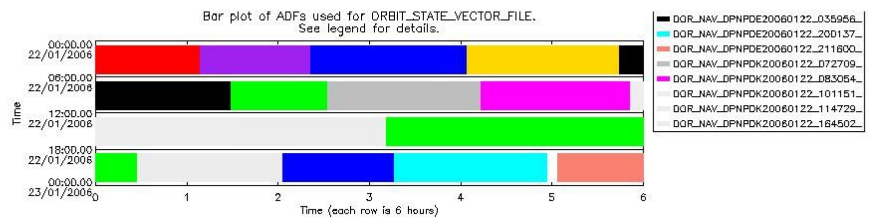
sciamachy_daily_report_level0_PFHS_5_35_N_20060122_6.PNG
