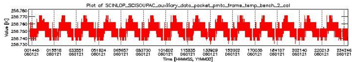
sciamachy_daily_report_level0_PFHS_5_35_N_20060121_1.PNG
