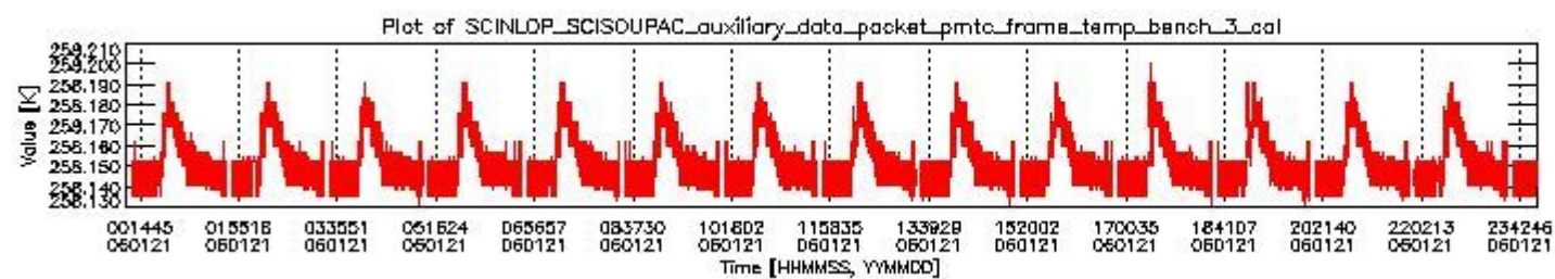
sciamachy_daily_report_level0_PFHS_5_35_N_20060121_2.PNG
