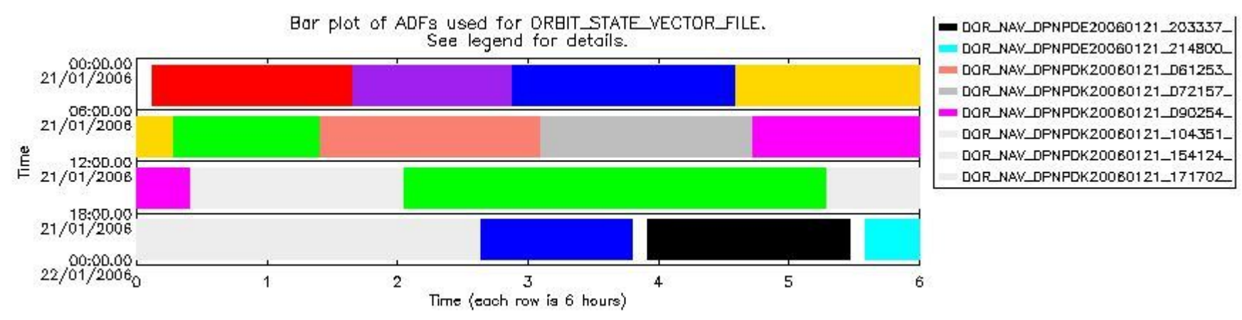
sciamachy_daily_report_level0_PFHS_5_35_N_20060121_6.PNG
