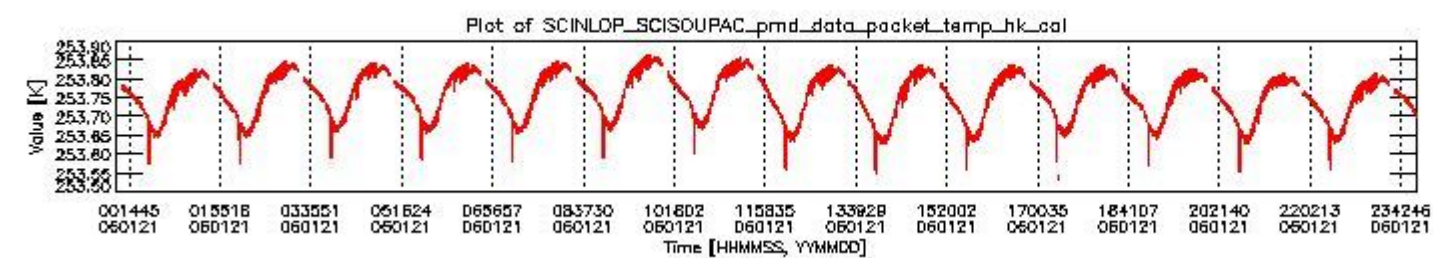
sciamachy_daily_report_level0_PFHS_5_35_N_20060121_3.PNG
