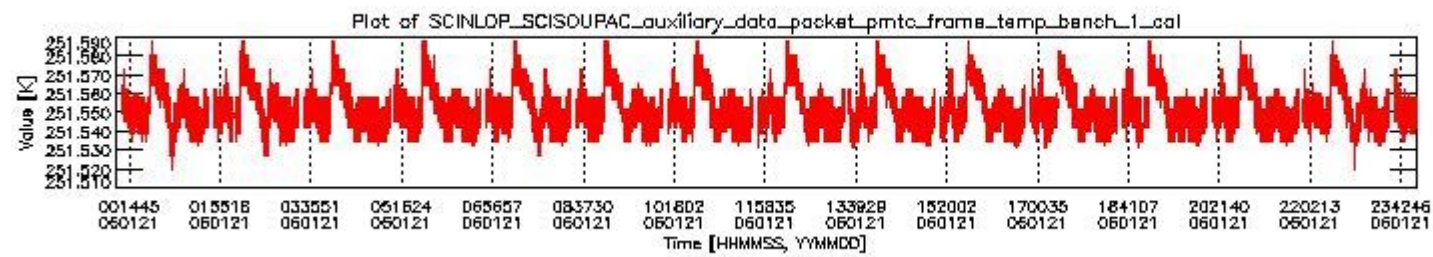
sciamachy_daily_report_level0_PFHS_5_35_N_20060121_0.PNG
